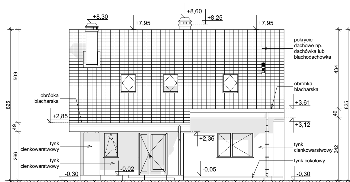
ELEWACJA FRONTOWA
