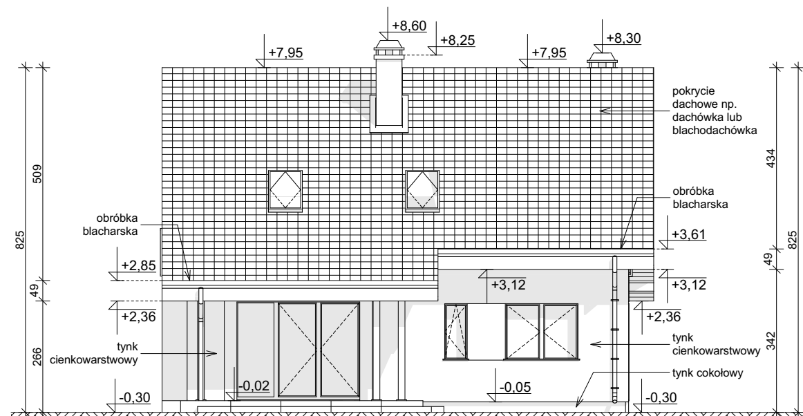
ELEWACJA OGRODOWA
