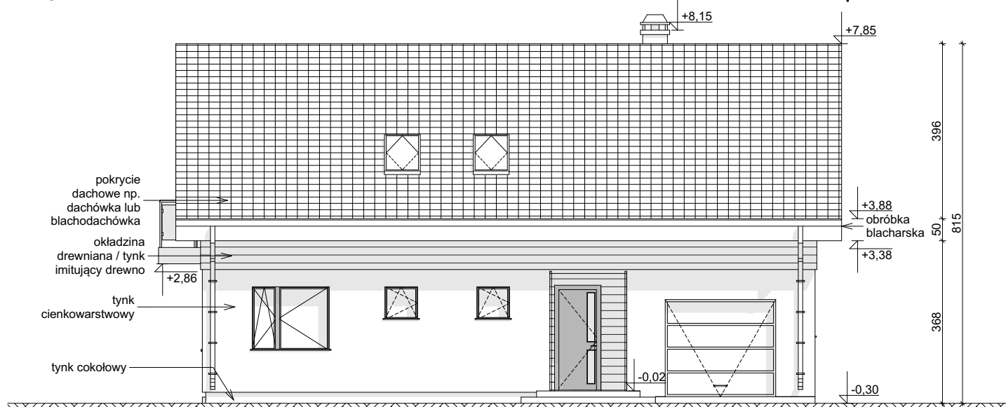
ELEWACJA FRONTOWA
