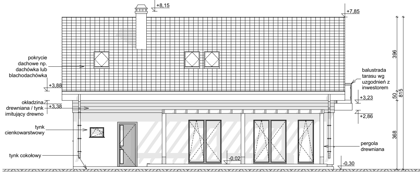
ELEWACJA OGRODOWA
