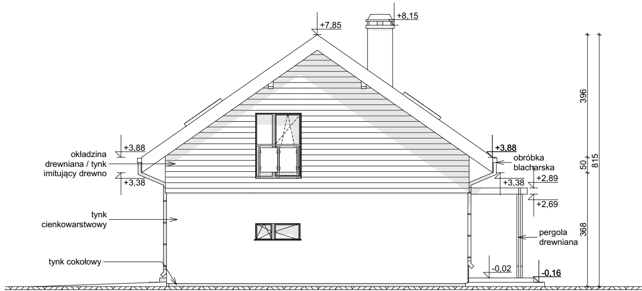
ELEWACJA BOCZNA
