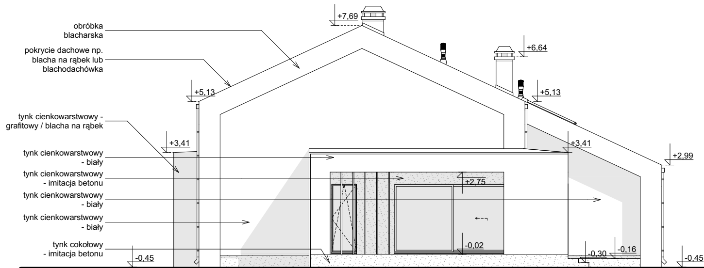
ELEWACJA OGRODOWA
