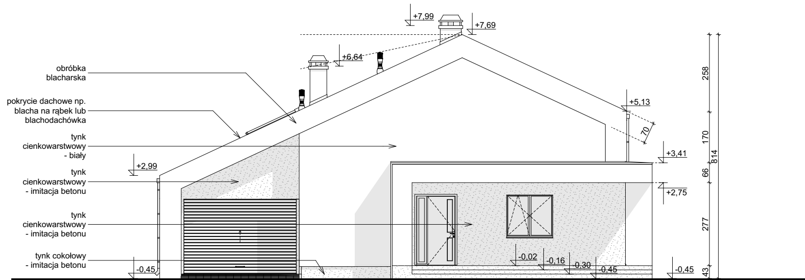
ELEWACJA FRONTOWA
