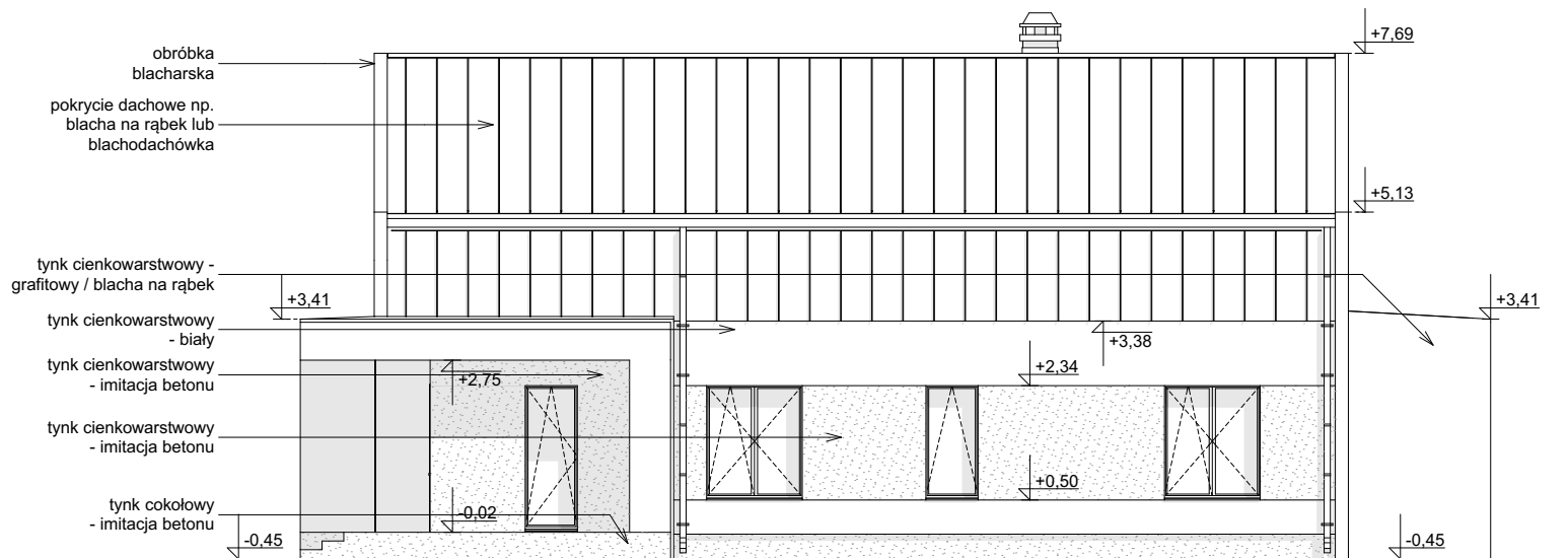
ELEWACJA BOCZNA
