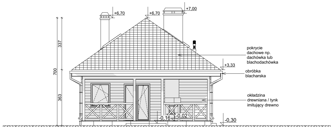
ELEWACJA OGRODOWA
