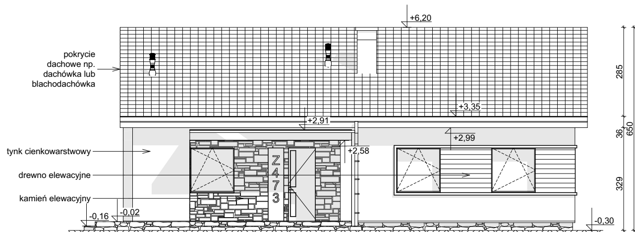
ELEWACJA FRONTOWA
