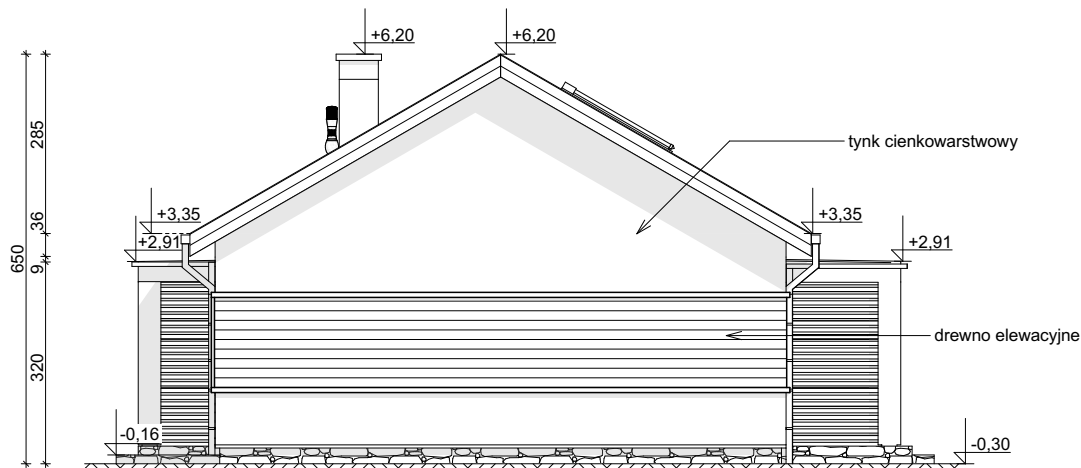
ELEWACJA BOCZNA
