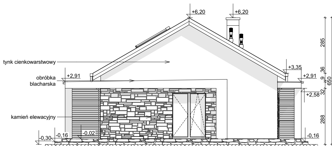
ELEWACJA BOCZNA
