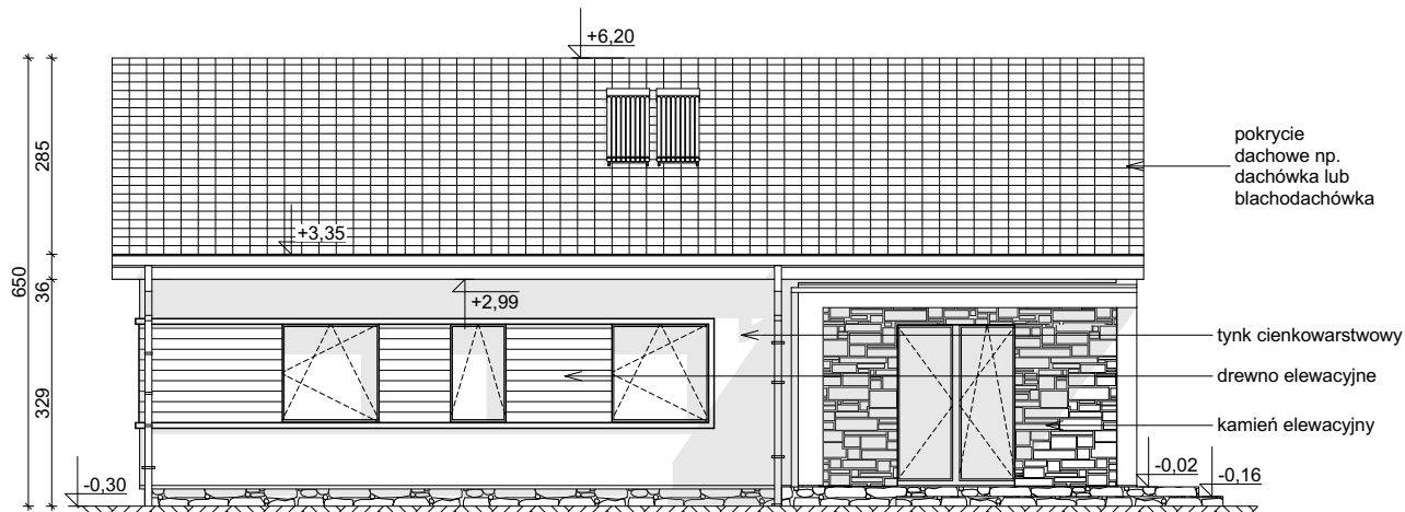
ELEWACJA OGRODOWA
