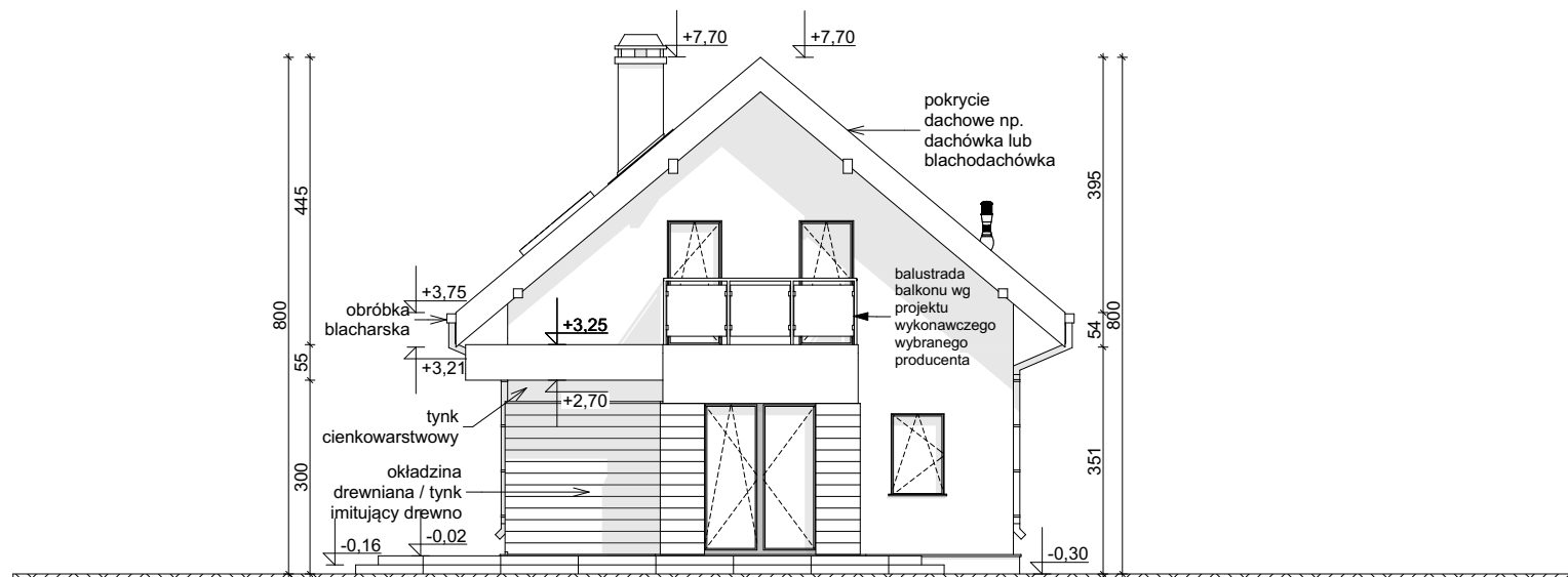
ELEWACJA OGRODOWA
