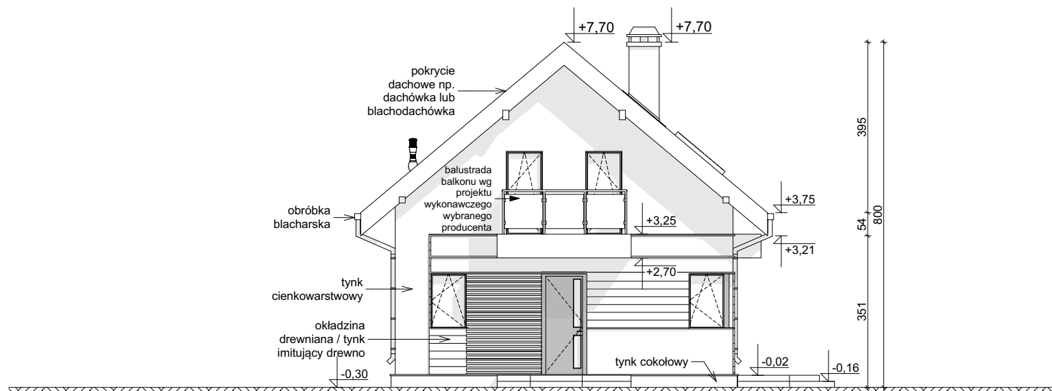
ELEWACJA FRONTOWA
