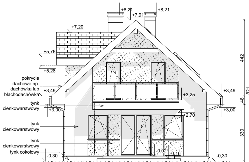
ELEWACJA OGRODOWA
