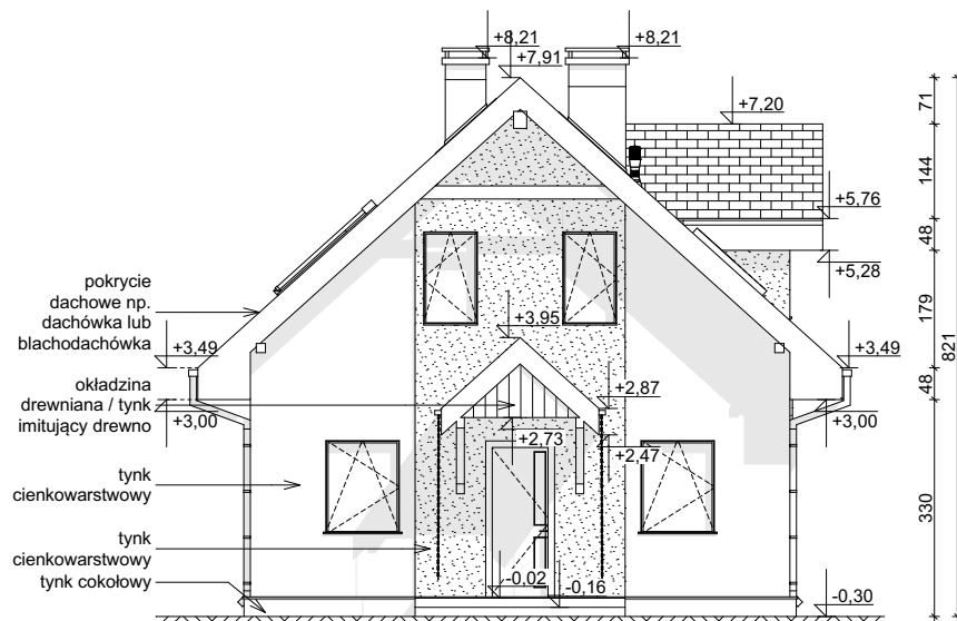
ELEWACJA FRONTOWA
