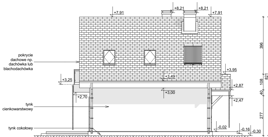
ELEWACJA BOCZNA
