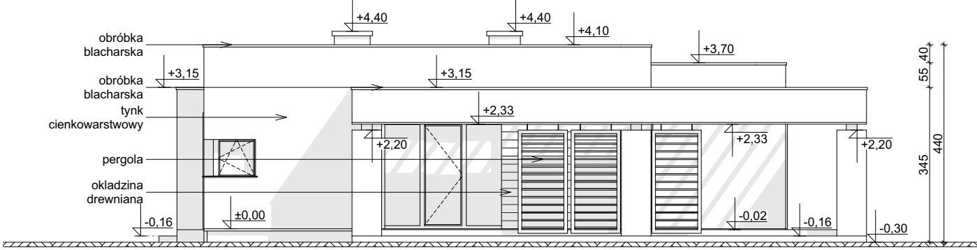
ELEWACJA BOCZNA
