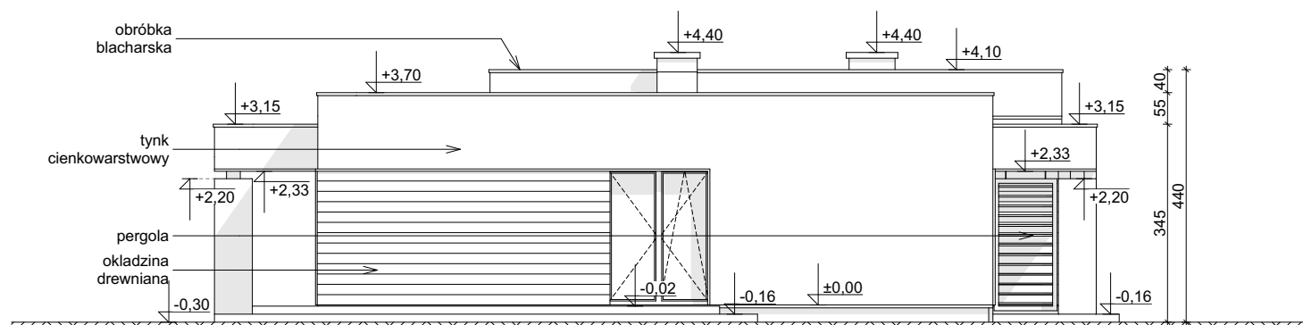
ELEWACJA BOCZNA
