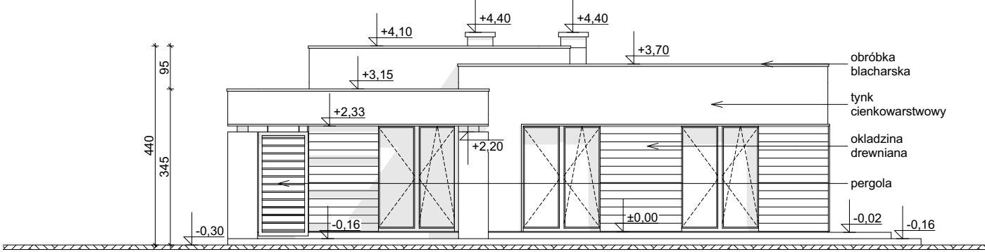
ELEWACJA OGRODOWA
