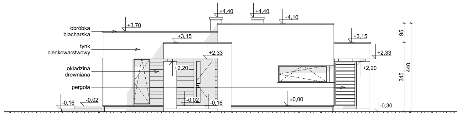
ELEWACJA FRONTOWA
