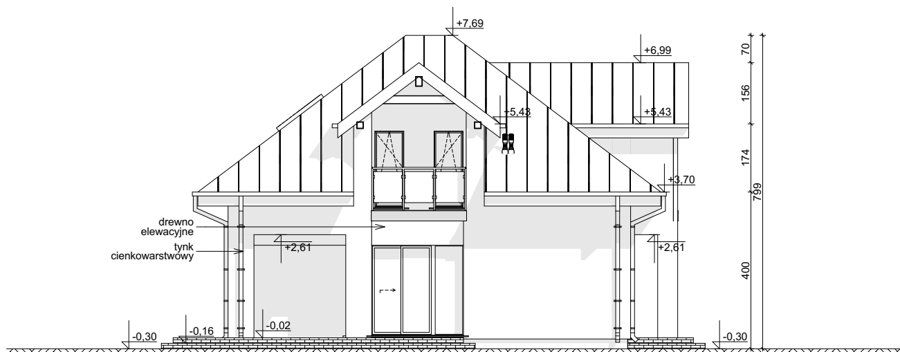
ELEWACJA BOCZNA
