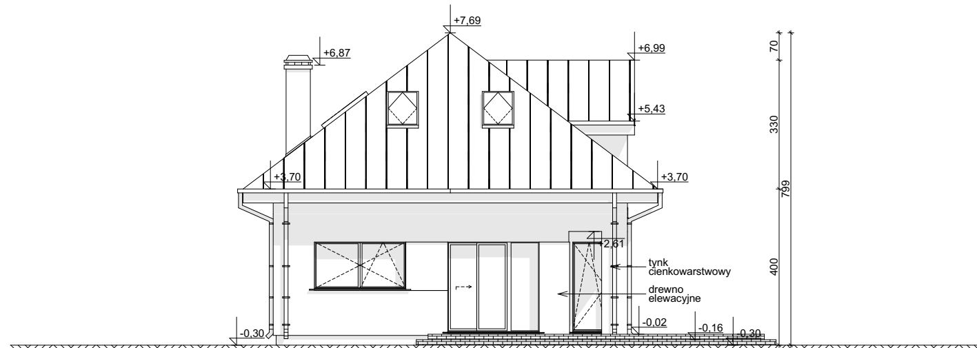
ELEWACJA OGRODOWA
