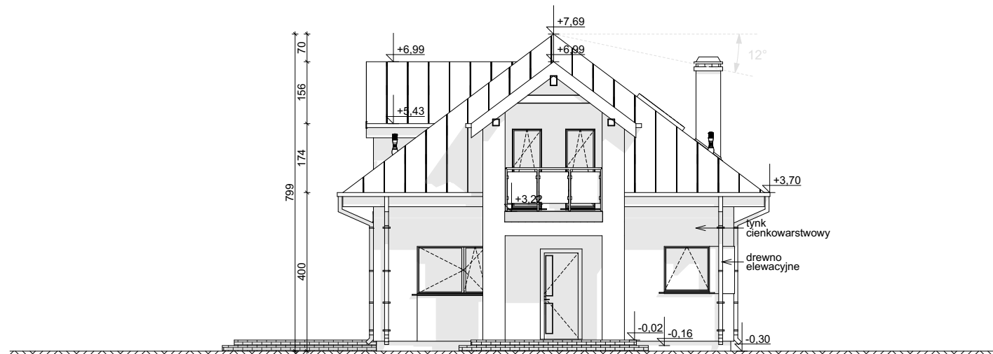
ELEWACJA FRONTOWA
