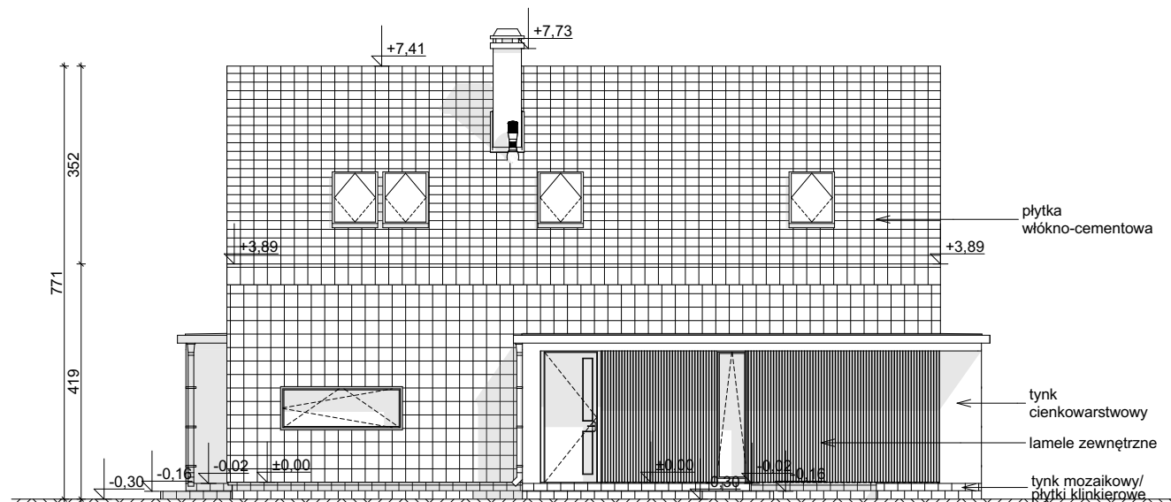
ELEWACJA FRONTOWA
