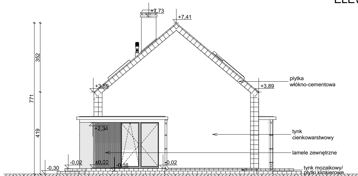
ELEWACJA BOCZNA
