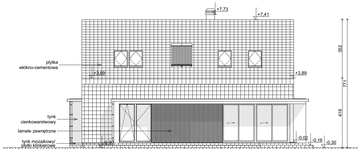
ELEWACJA OGRODOWA
