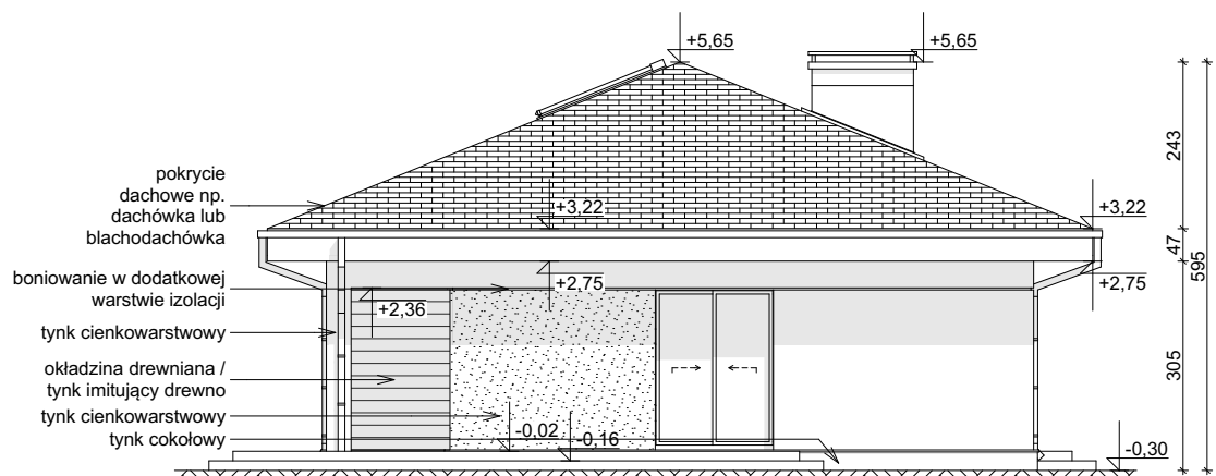
ELEWACJA BOCZNA
