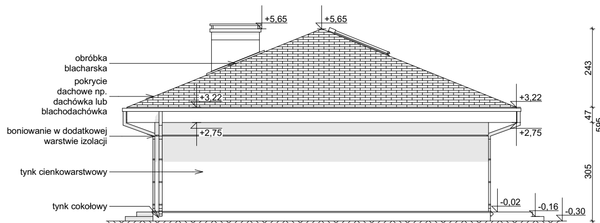
ELEWACJA BOCZNA
