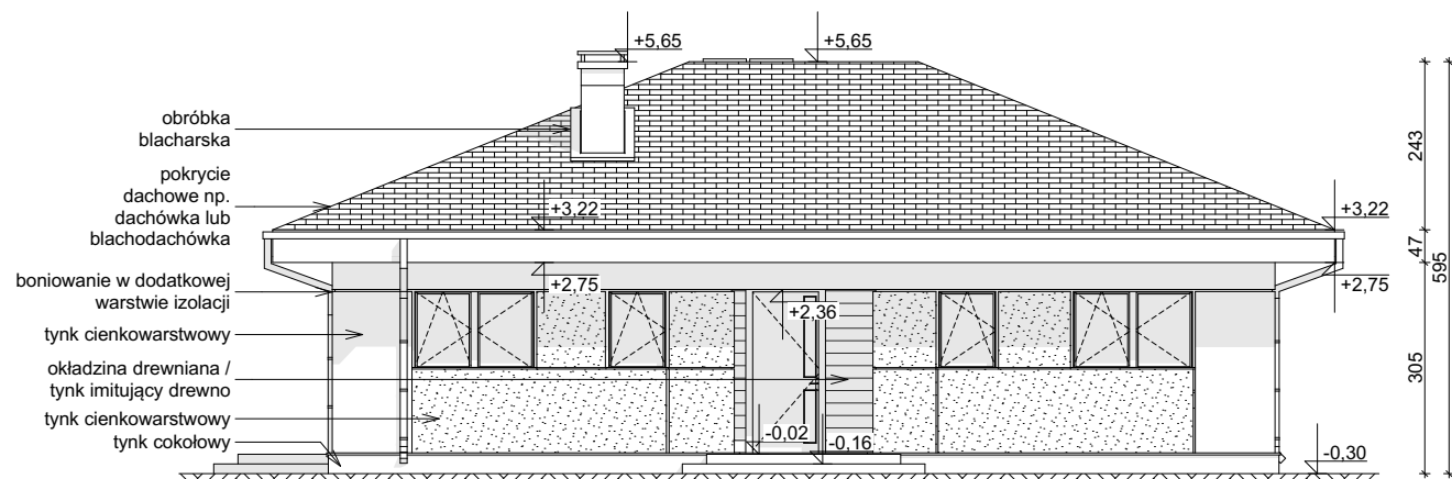
ELEWACJA FRONTOWA
