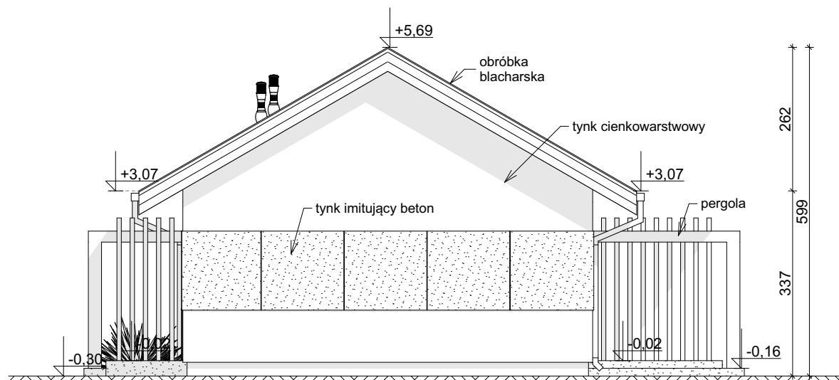
ELEWACJA BOCZNA
