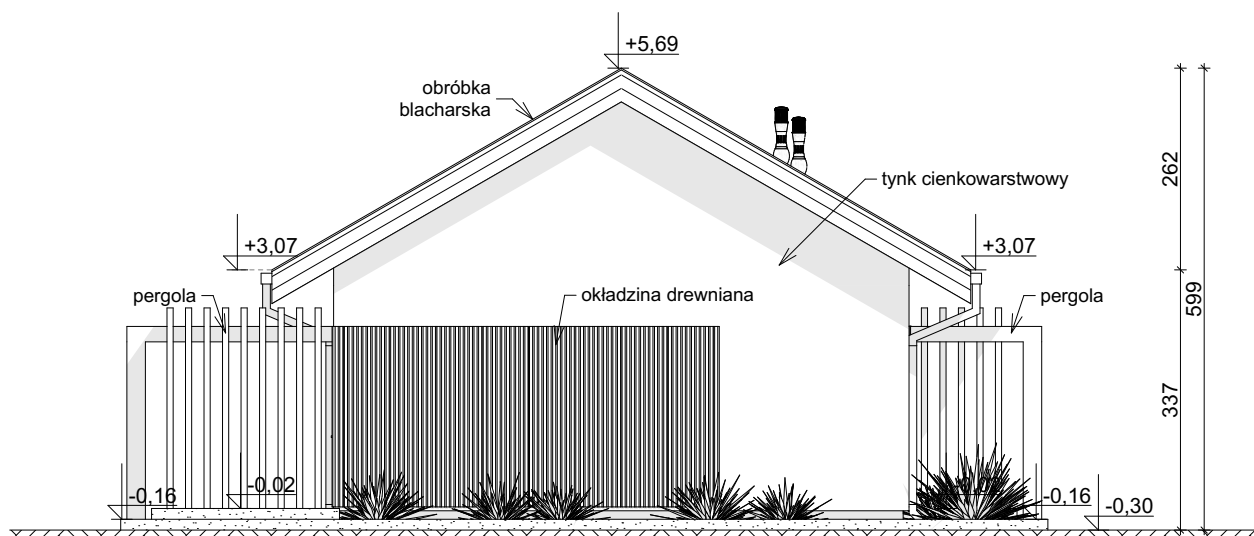
ELEWACJA BOCZNA
