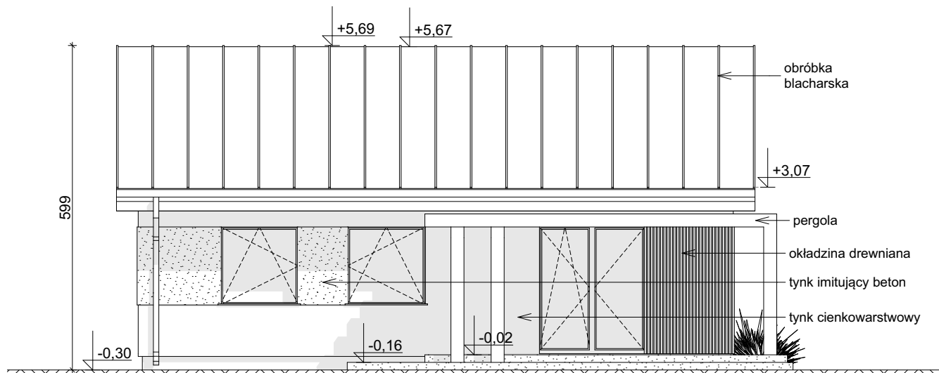
ELEWACJA OGRODOWA
