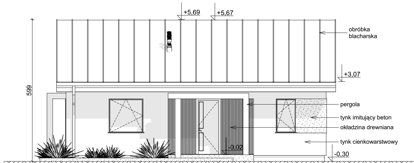
ELEWACJA FRONTOWA
