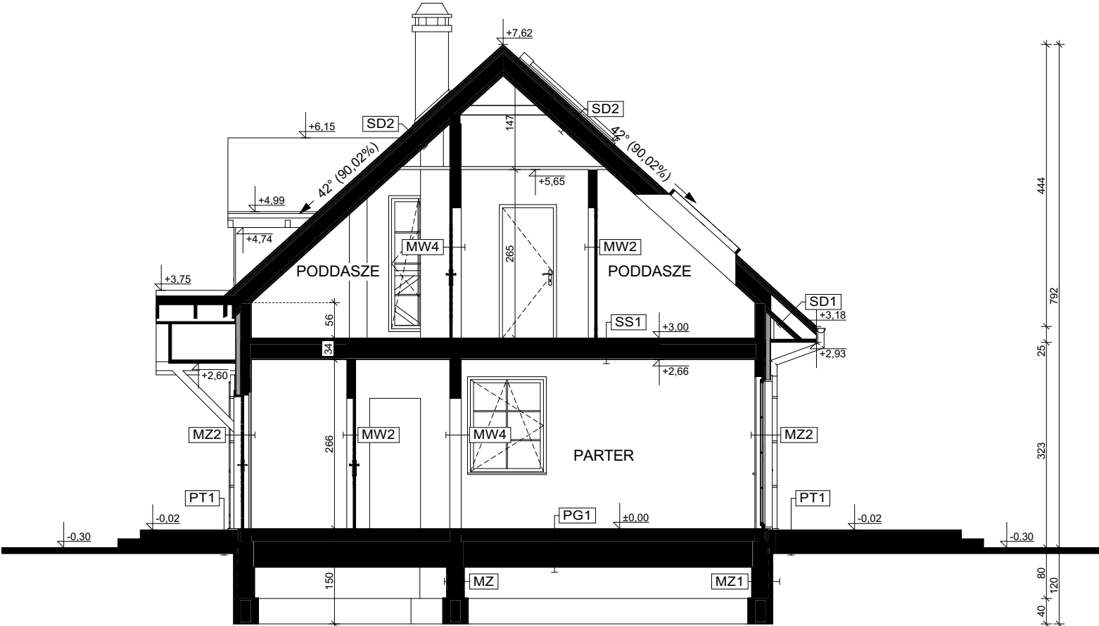
PRZEKRÓJ B-B
