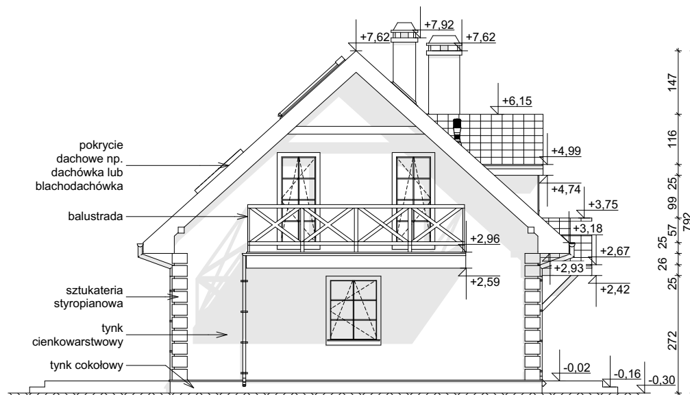
ELEWACJA BOCZNA
