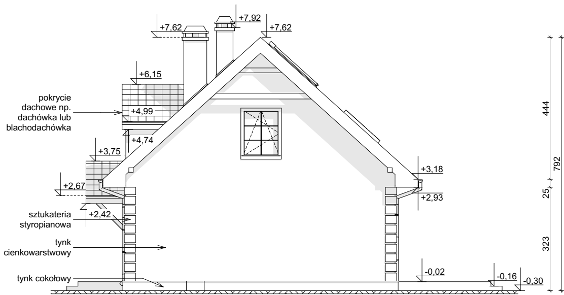
ELEWACJA BOCZNA
