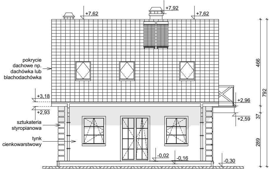
ELEWACJA OGRODOWA
