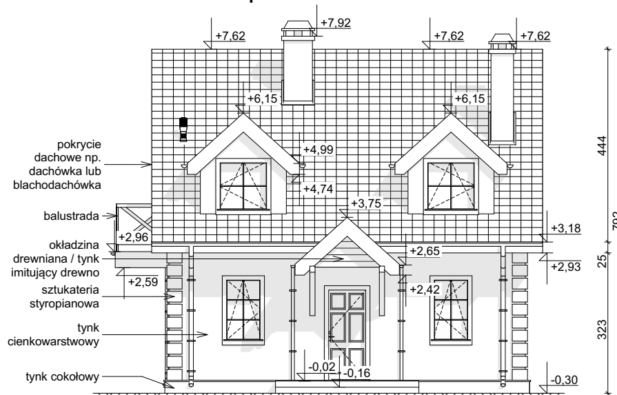
ELEWACJA FRONTOWA
