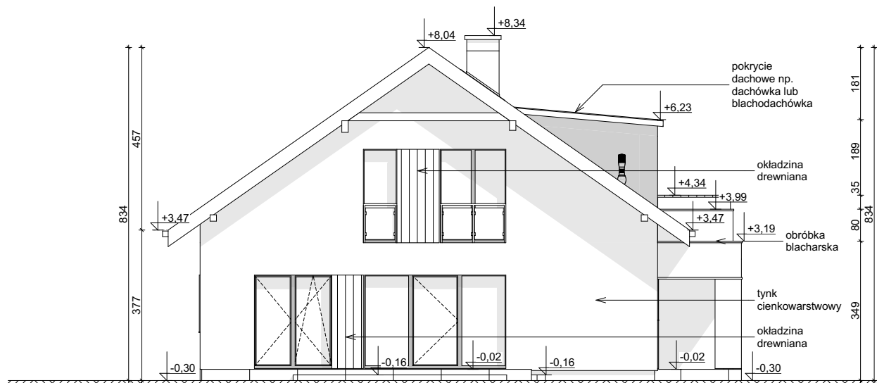
ELEWACJA BOCZNA
