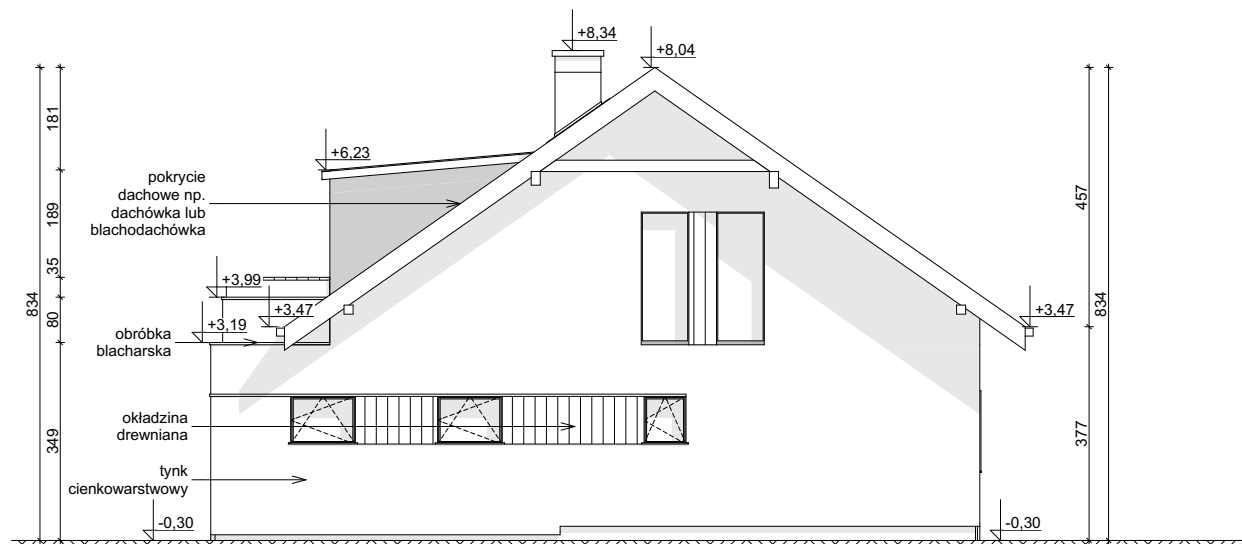
ELEWACJA BOCZNA
