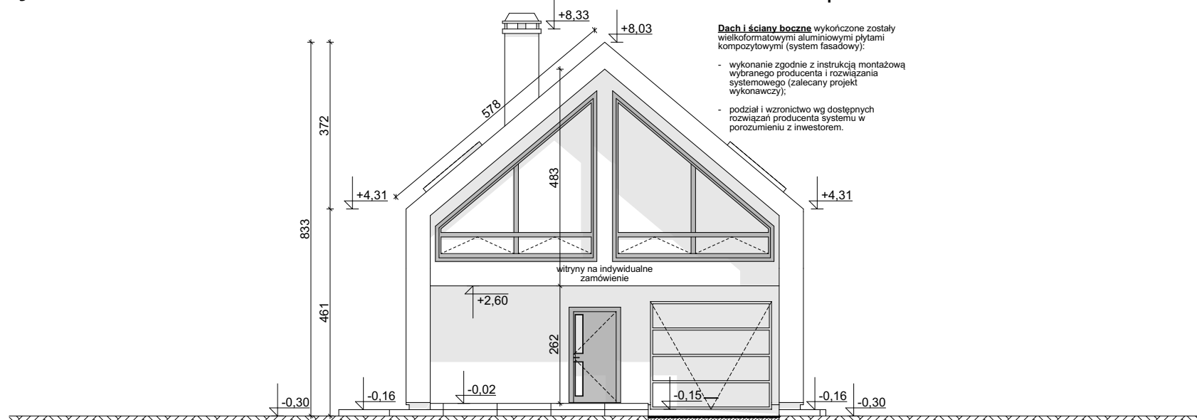
ELEWACJA FRONTOWA
