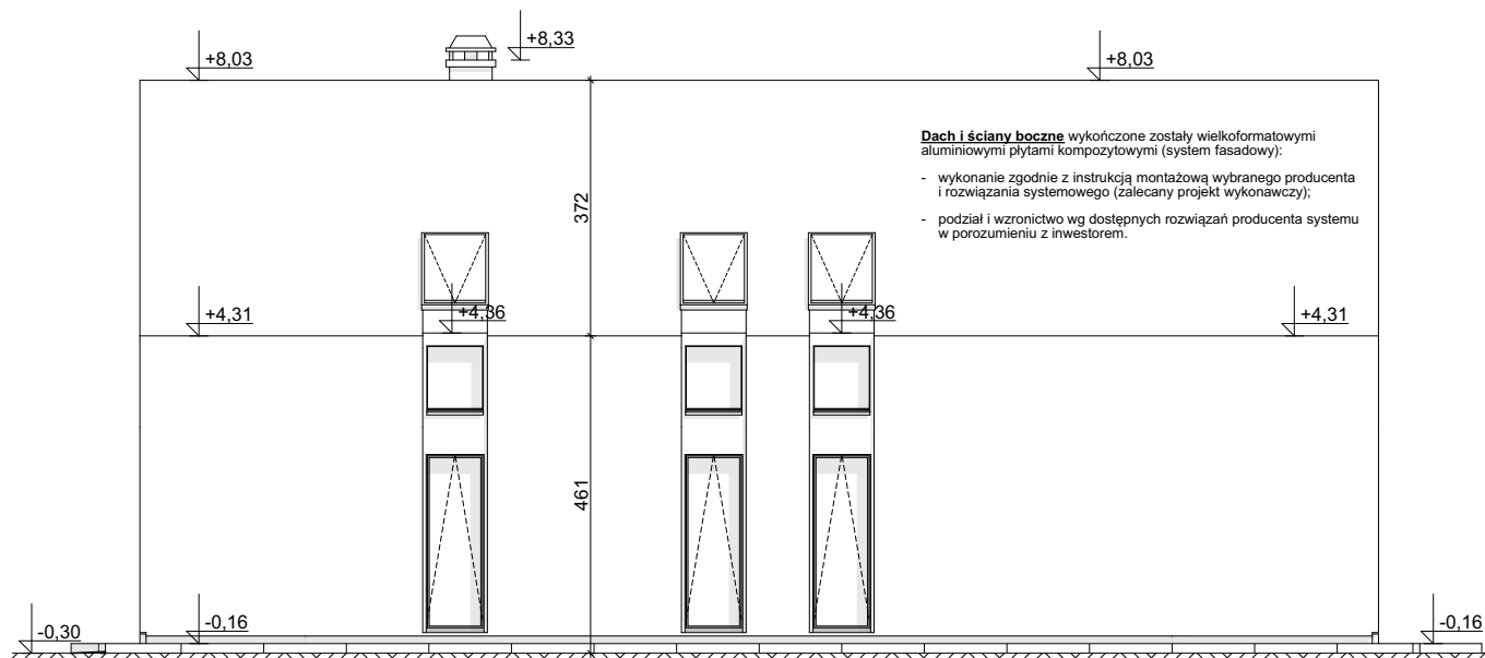
ELEVACJA BOCZNA
