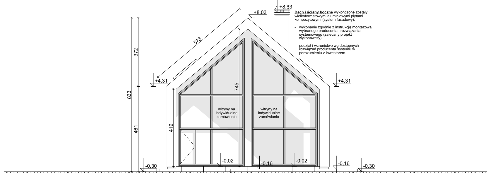
ELEVACJA OGRODOWA
