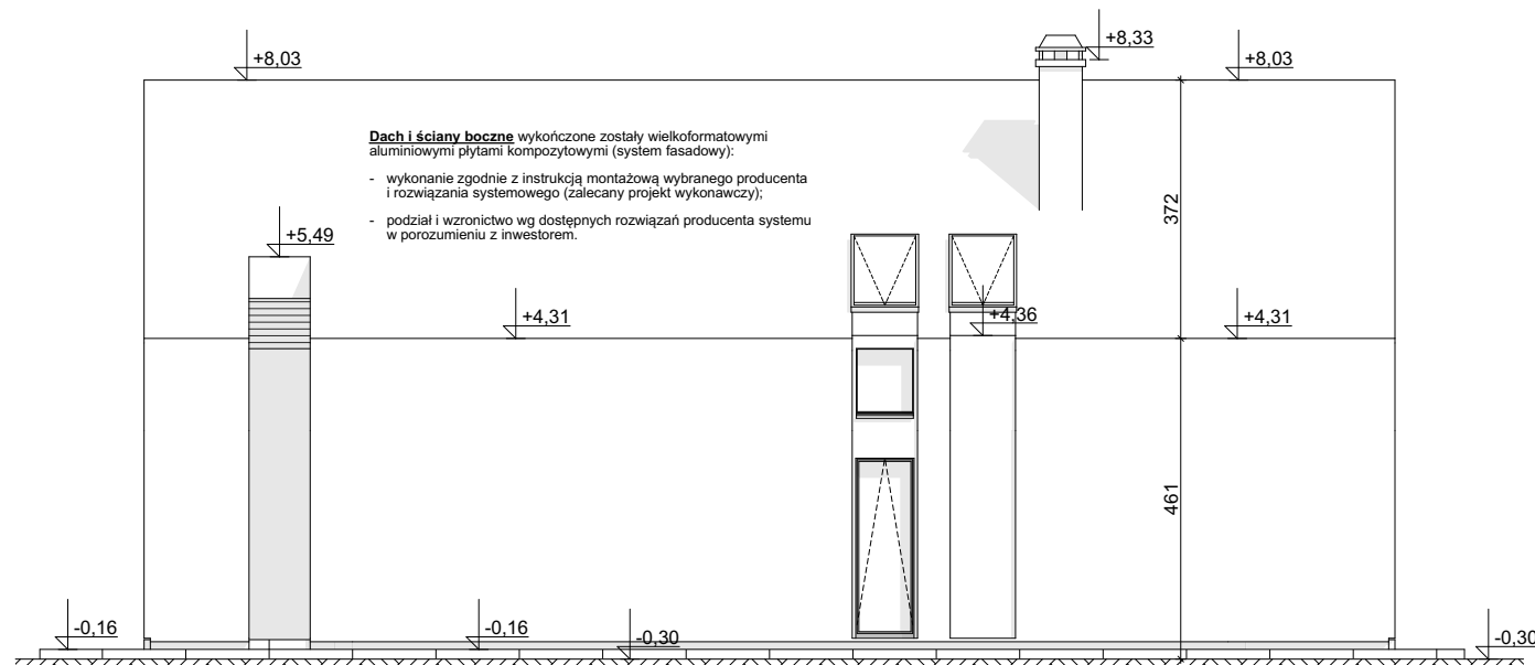
ELEWACJA BOCZNA
