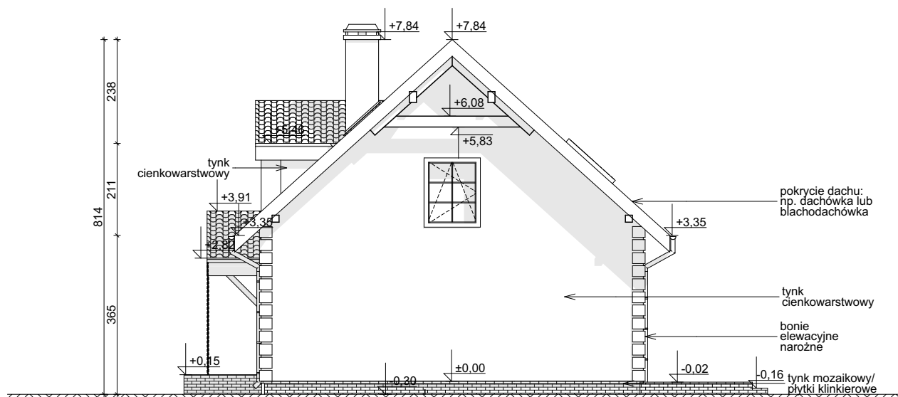
ELEWACJA BOCZNA
