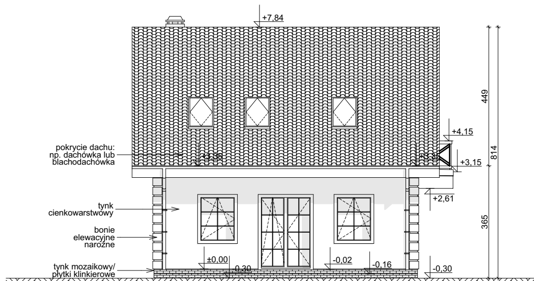
ELEWACJA OGRODOWA
