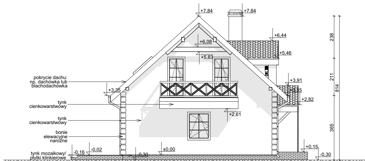
ELEWACJA BOCZNA
