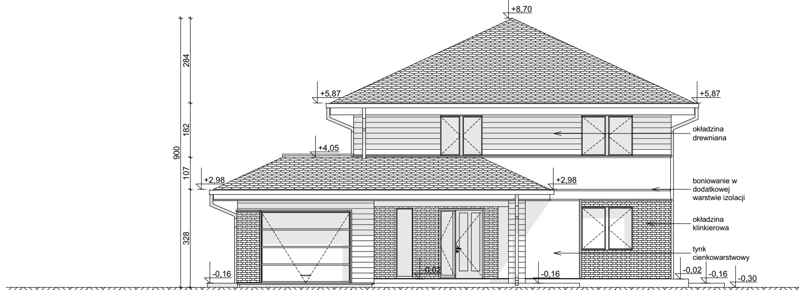
ELEWACJA FRONTOWA
