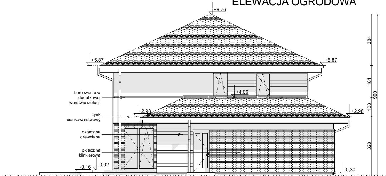
ELEWACJA BOCZNA
