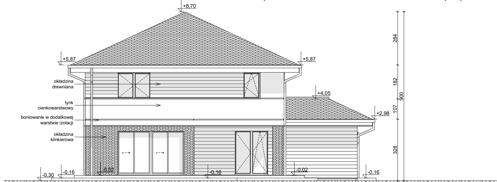
ELEWACJA OGRODOWA
