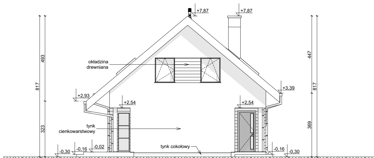
ELEWACJA BOCZNA
