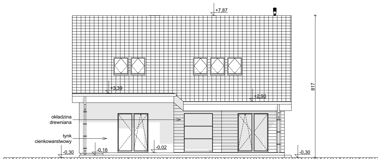
ELEWACJA OGRODOWA
