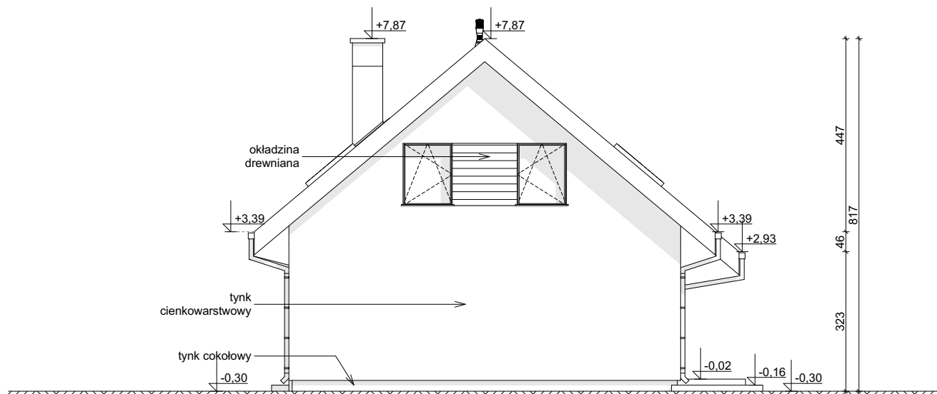
ELEWACJA BOCZNA
