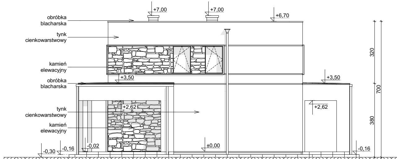
ELEWACJA BOCZNA
