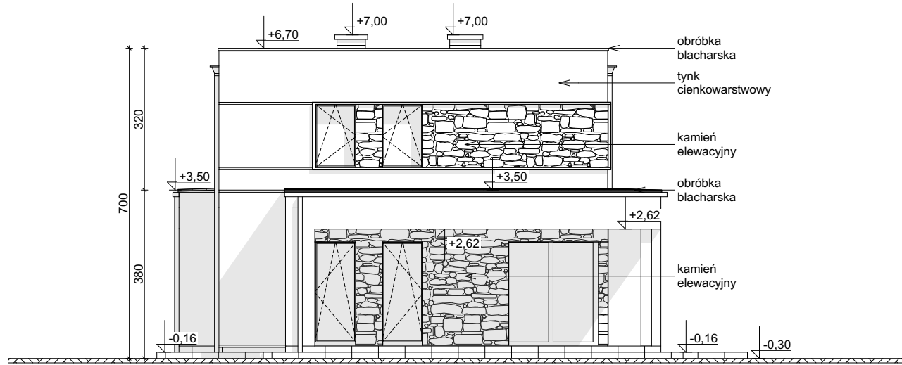
ELEWACJA OGRODOWA
