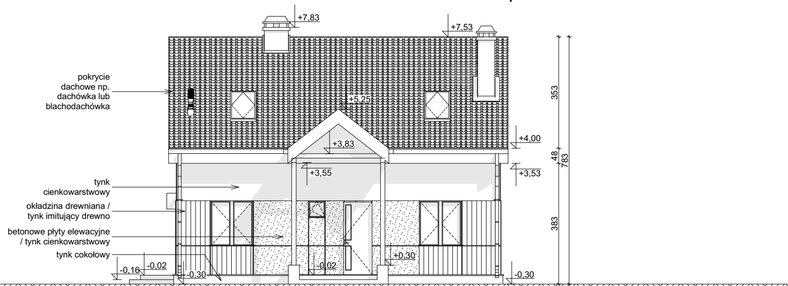
ELEWACJA FRONTOWA
