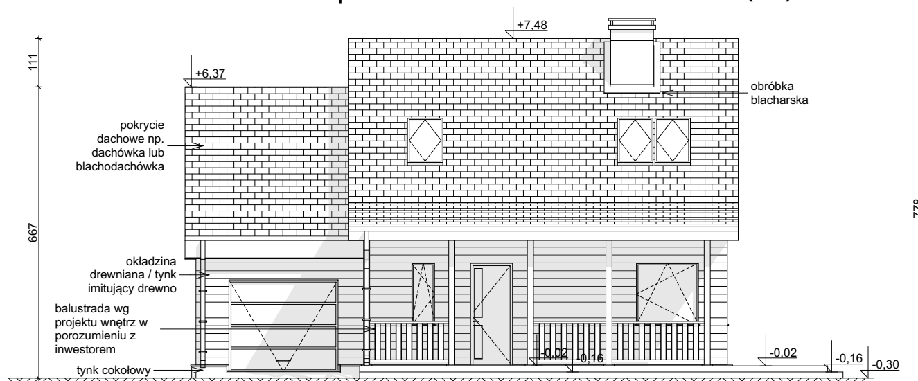
ELEWACJA FRONTOWA
