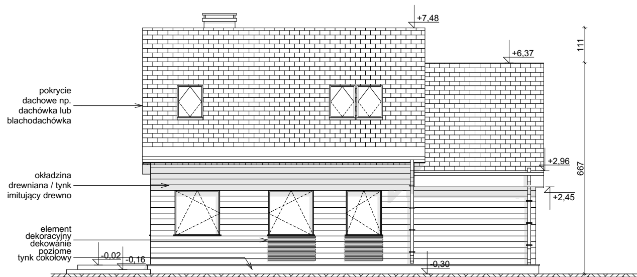
ELEWACJA OGRODOWA
