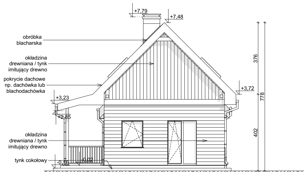
ELEWACJA BOCZNA
