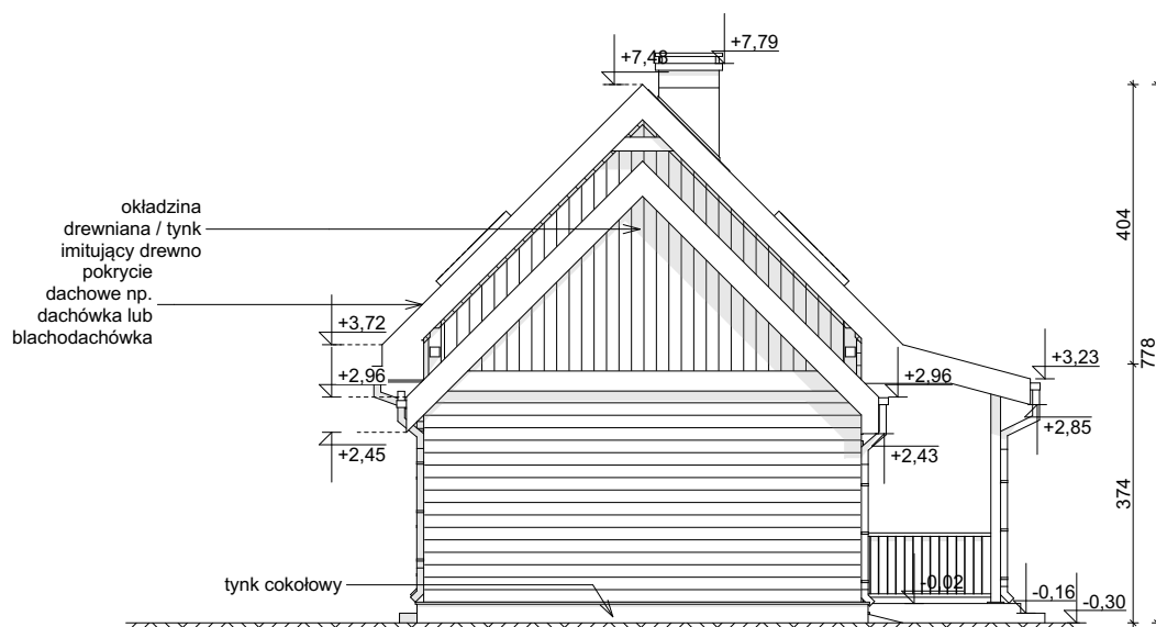
ELEWACJA BOCZNA
