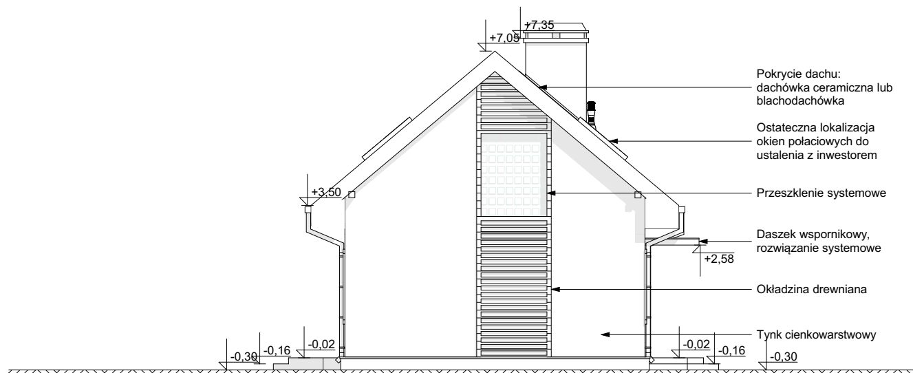
ELEWACJA BOCZNA
