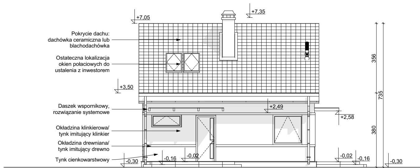
ELEWACJA FRONTOWA
