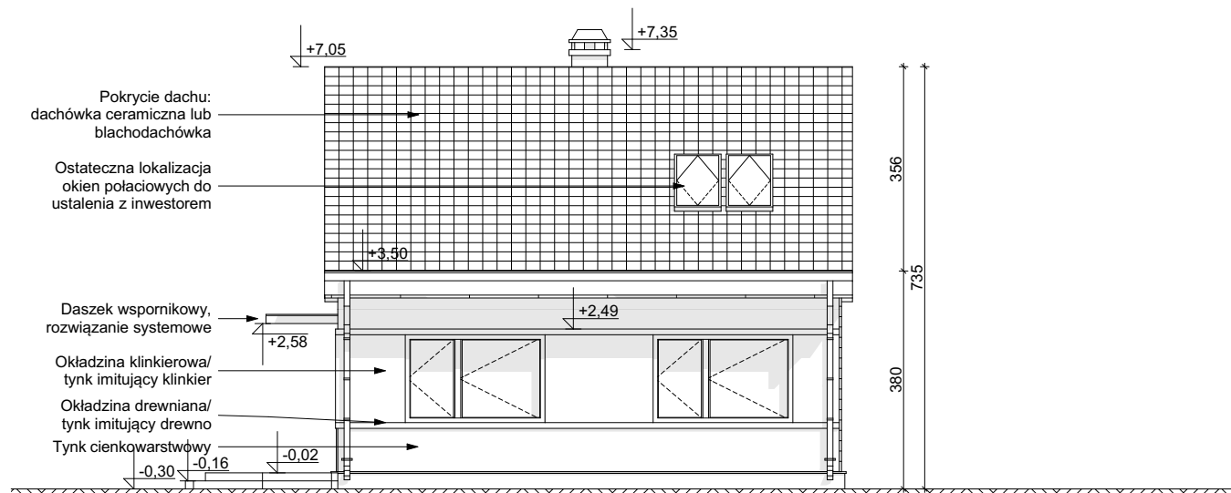
ELEWACJA OGRODOWA
