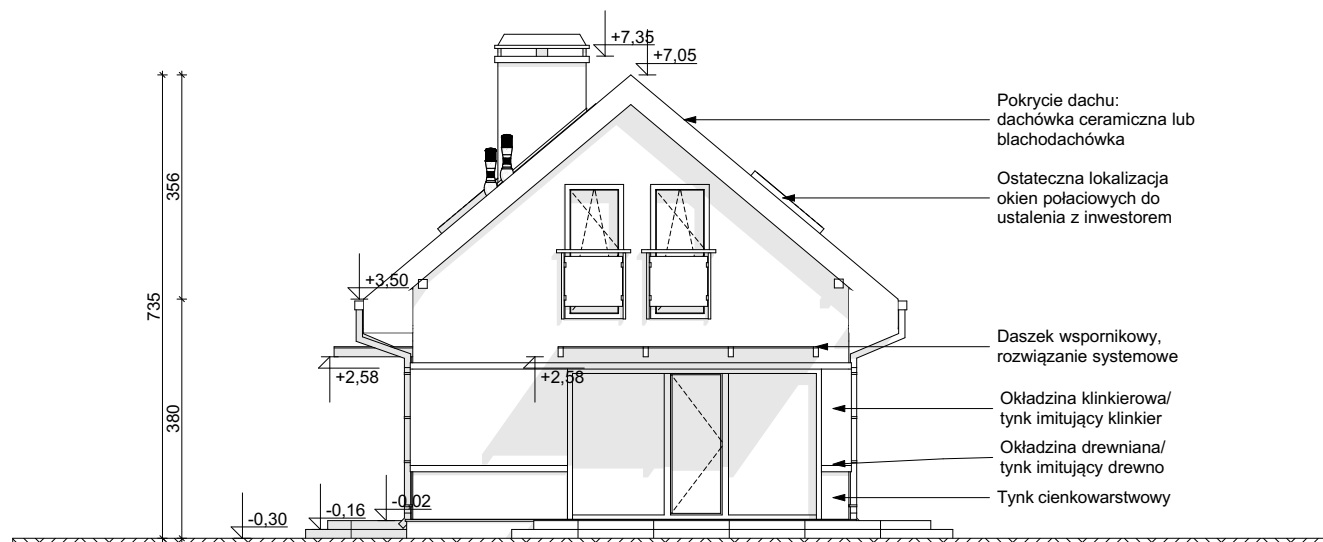
ELEWACJA BOCZNA
