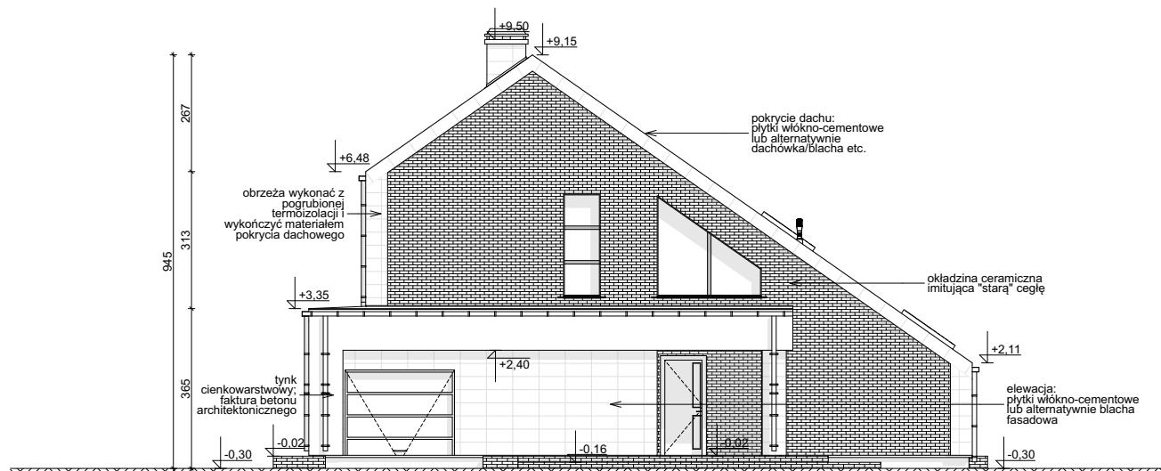
ELEWACJA FRONTOWA
