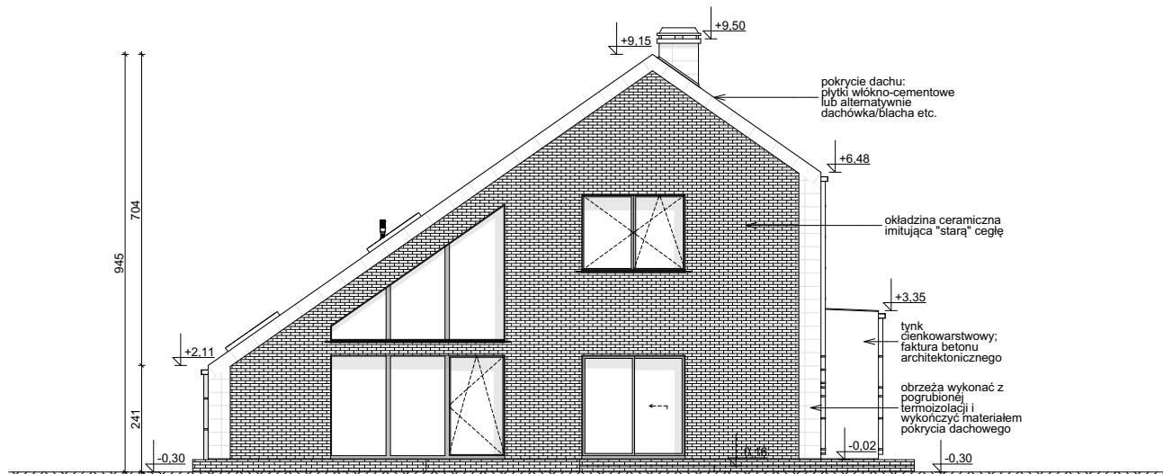
ELEWACJA OGRODOWA
