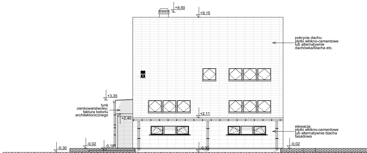
ELEWACJA BOCZNA
