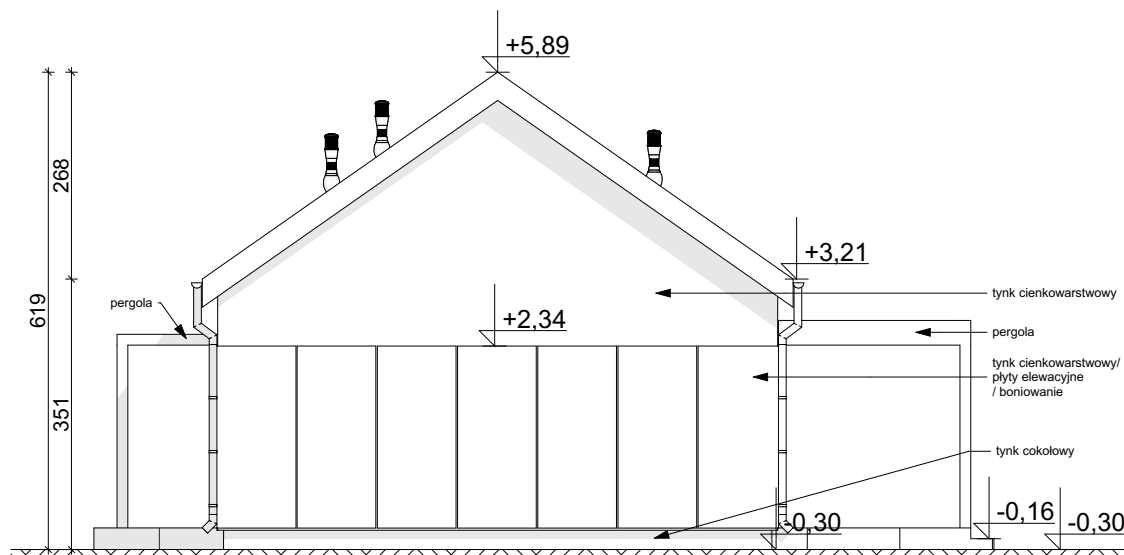
ELEWACJA BOCZNA
