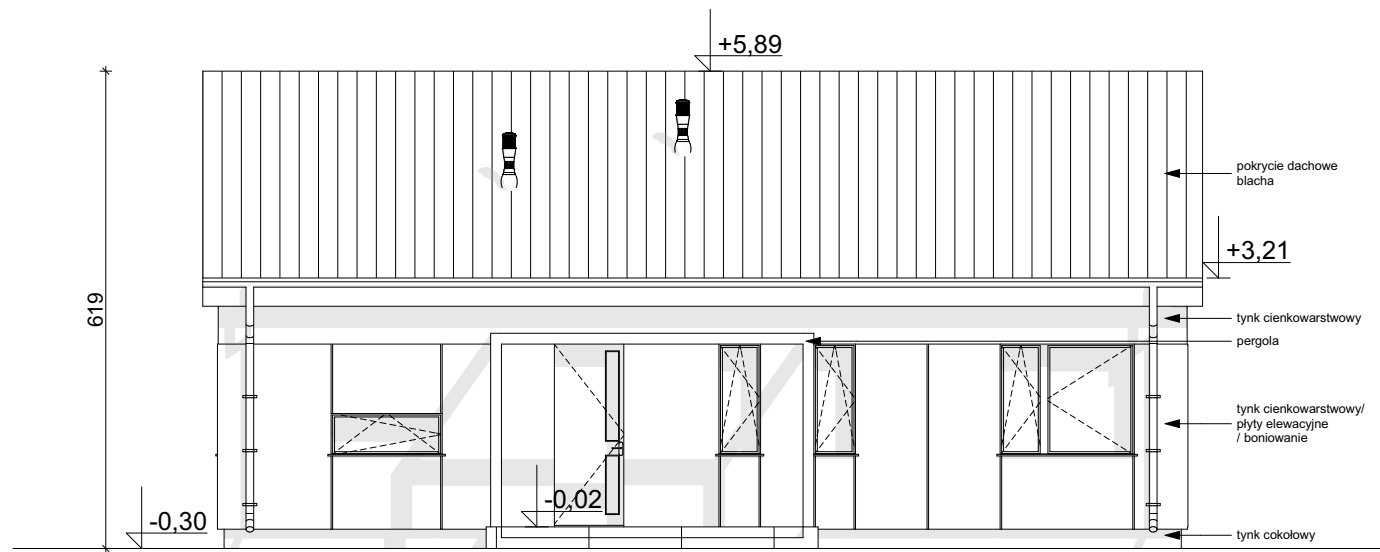
ELEWACJA FRONTOWA
