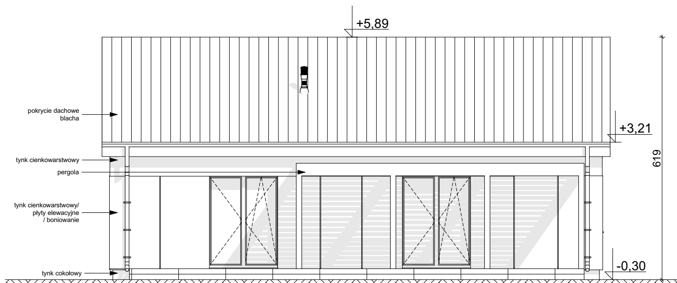
ELEWACJA OGRODOWA
