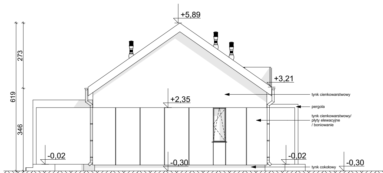
ELEWACJA BOCZNA
