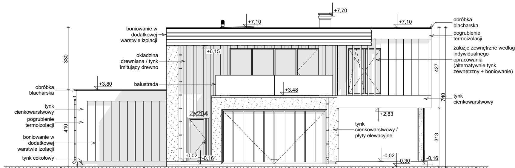
ELEWACJA FRONTOWA
