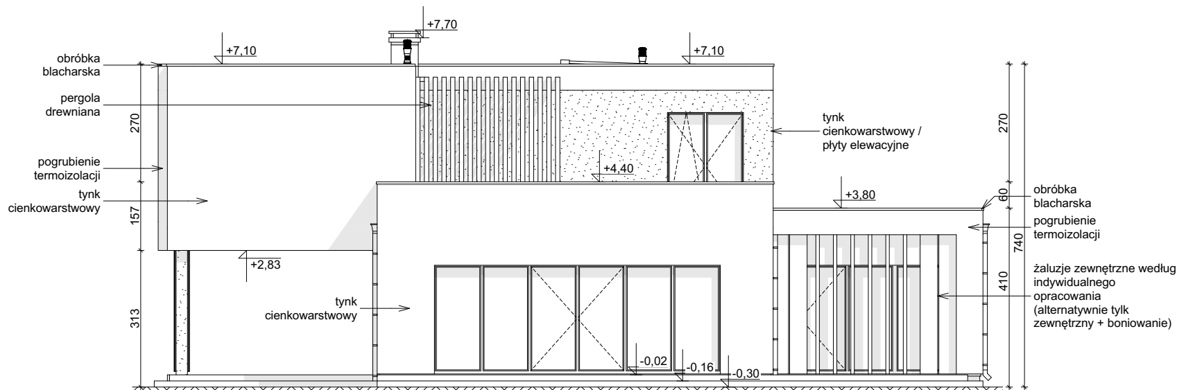
ELEWACJA OGRODOWA
