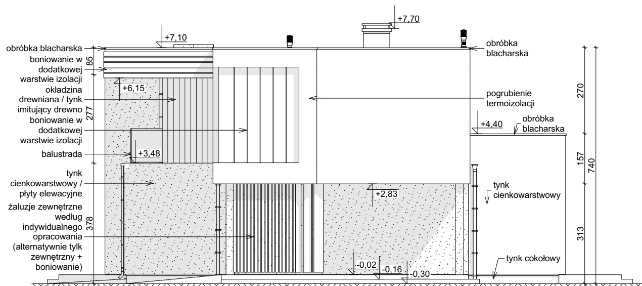
ELEWACJA BOCZNA
