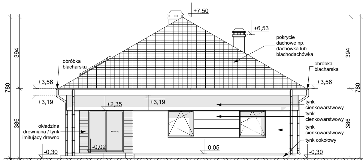
ELEWACJA OGRODOWA
