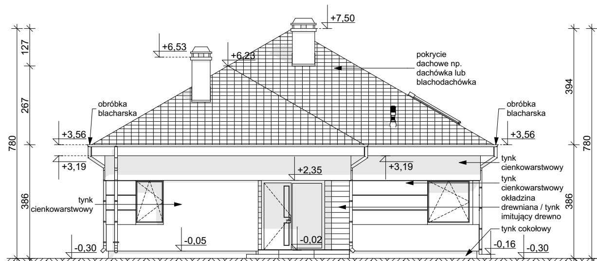
ELEWACJA FRONTOWA
