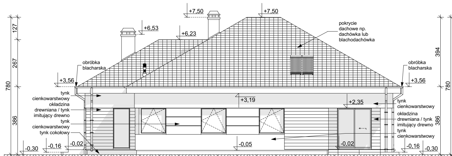
ELEWACJA BOCZNA
