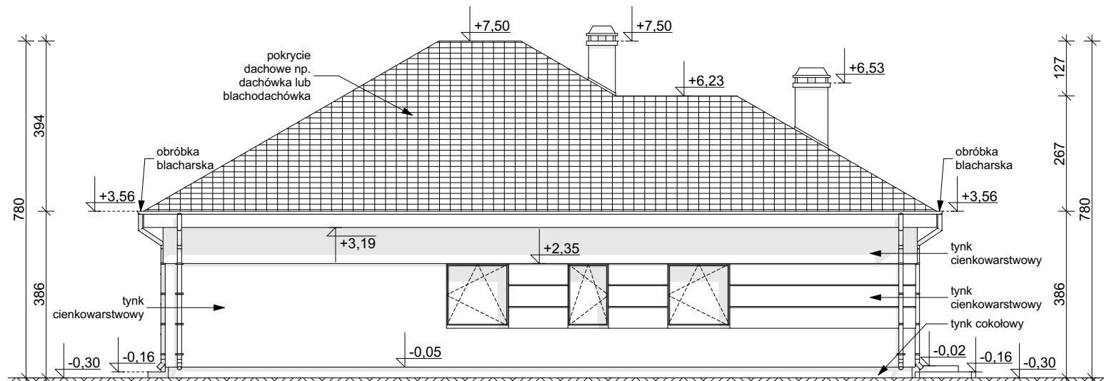
ELEWACJA BOCZNA
