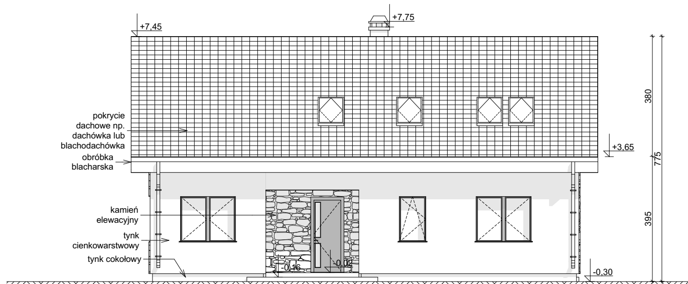
ELEWACJA FRONTOWA
