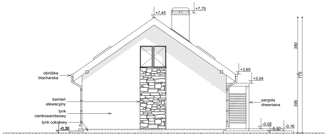
ELEWACJA BOCZNA
