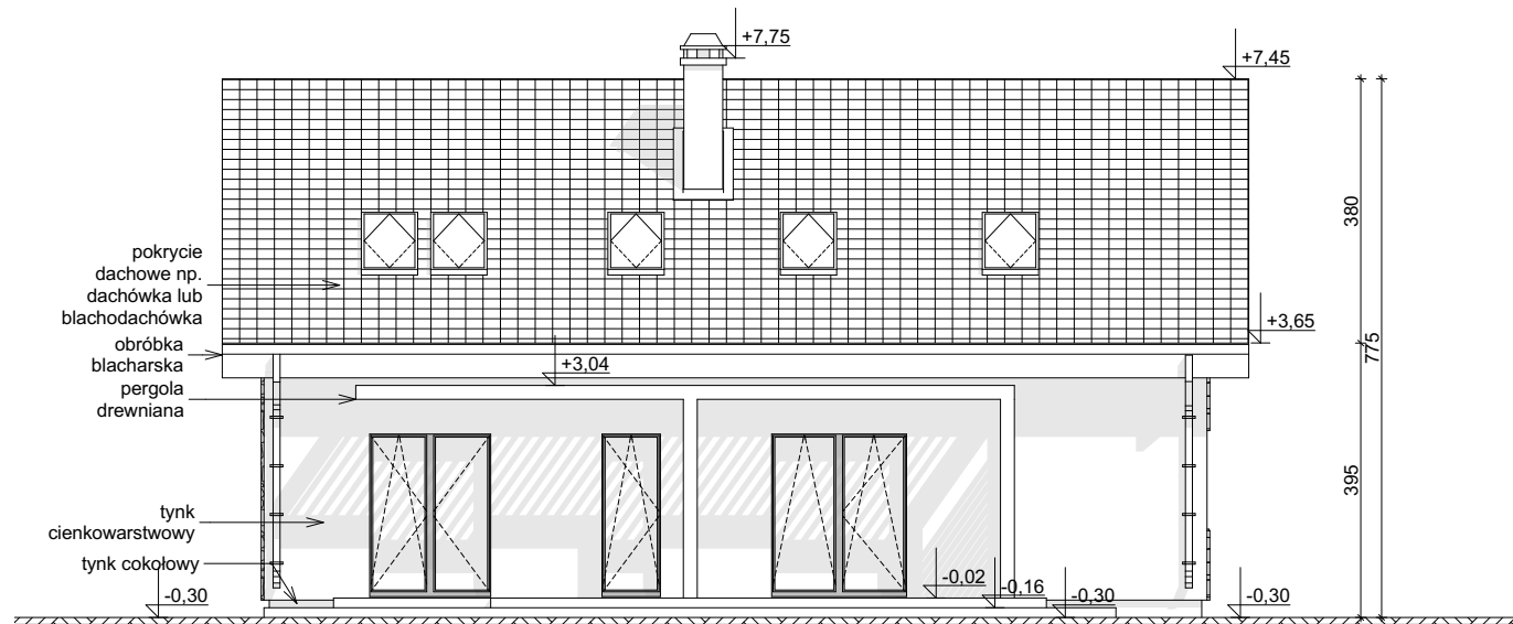
ELEWACJA OGRODOWA
