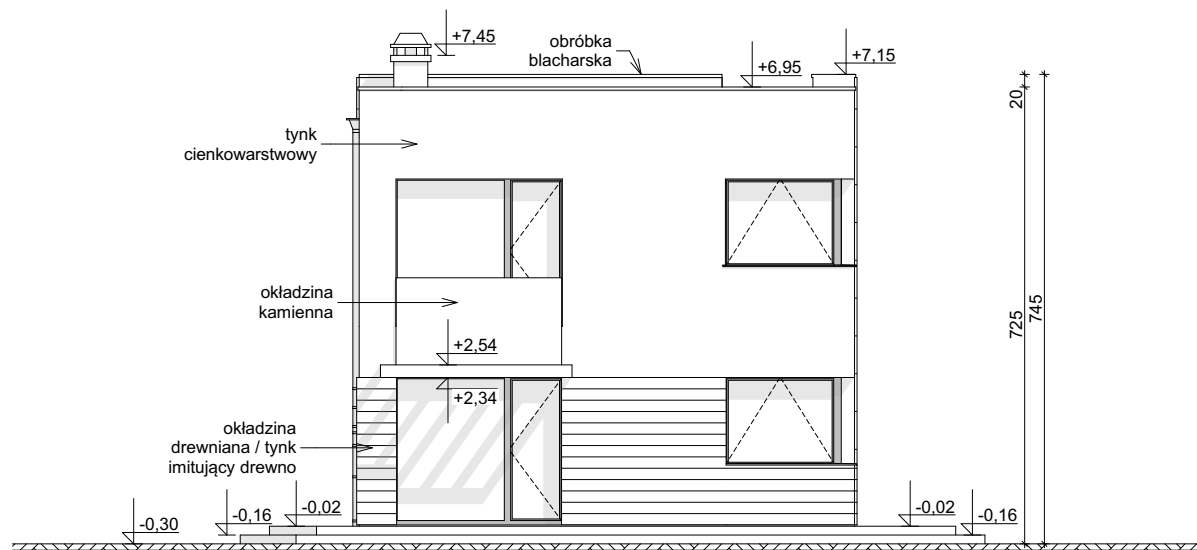
ELEWACJA OGRODOWA
