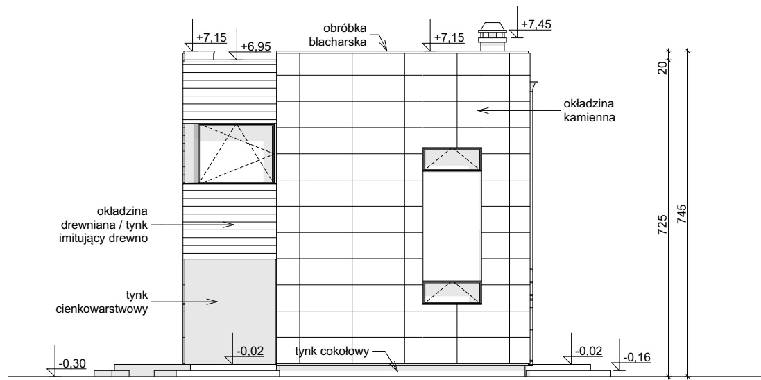
ELEWACJA FRONTOWA
