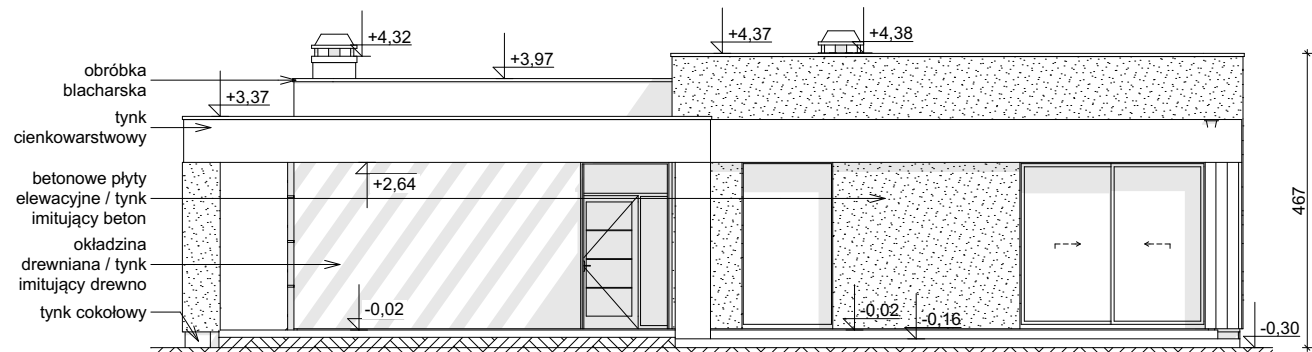
ELEWACJA FRONTOWA
