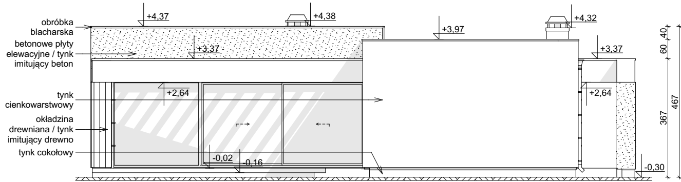
ELEWACJA OGRODOWA
