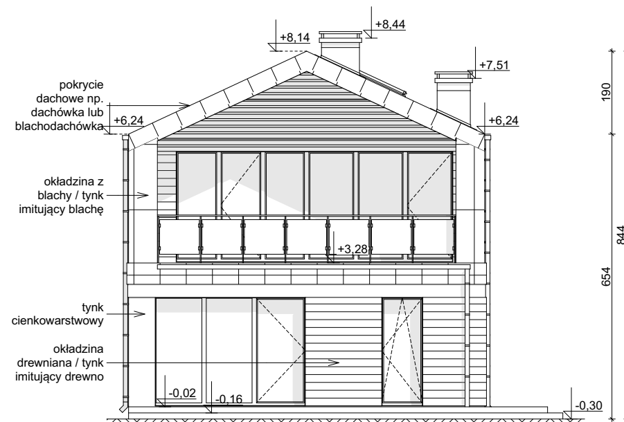
ELEWACJA OGRODOWA
