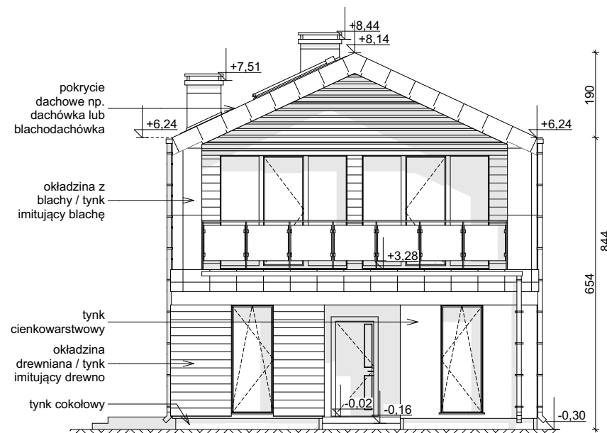
ELEWACJA FRONTOWA
