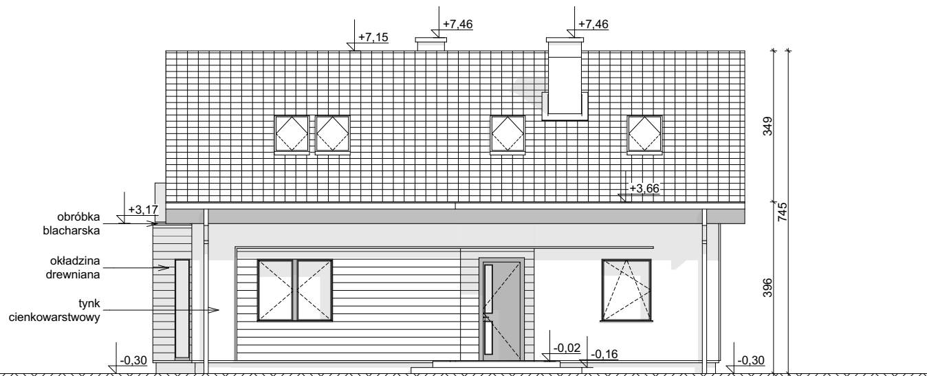
ELEWACJA FRONTOWA
