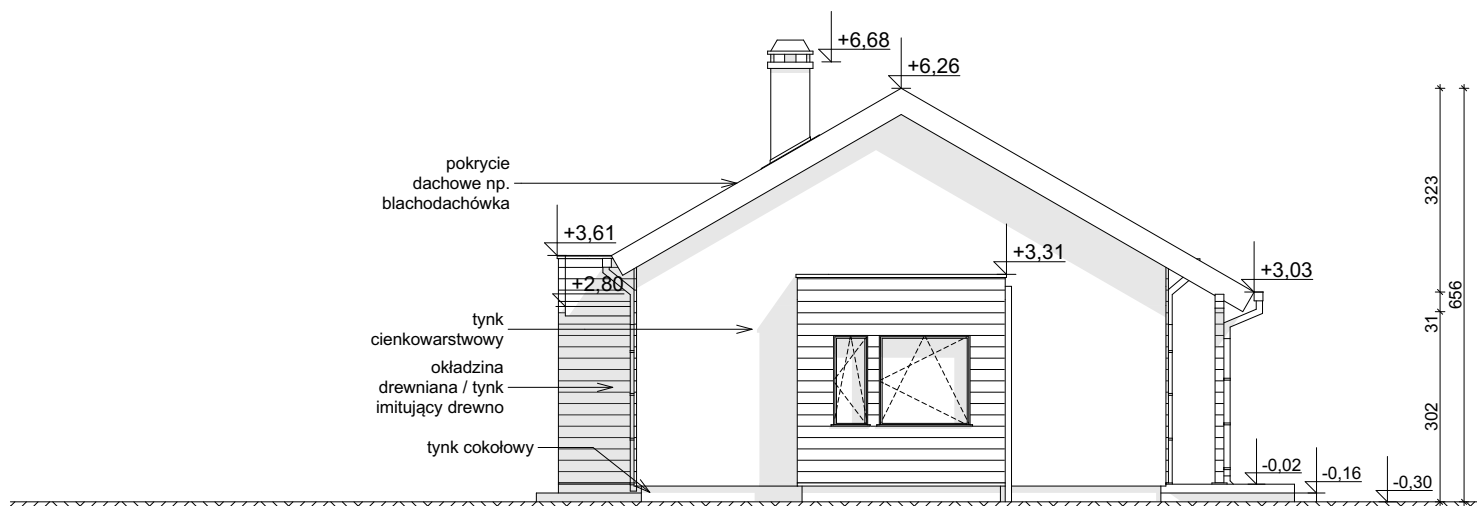
ELEWACJA BOCZNA
