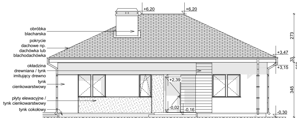
ELEWACJA FRONTOWA
