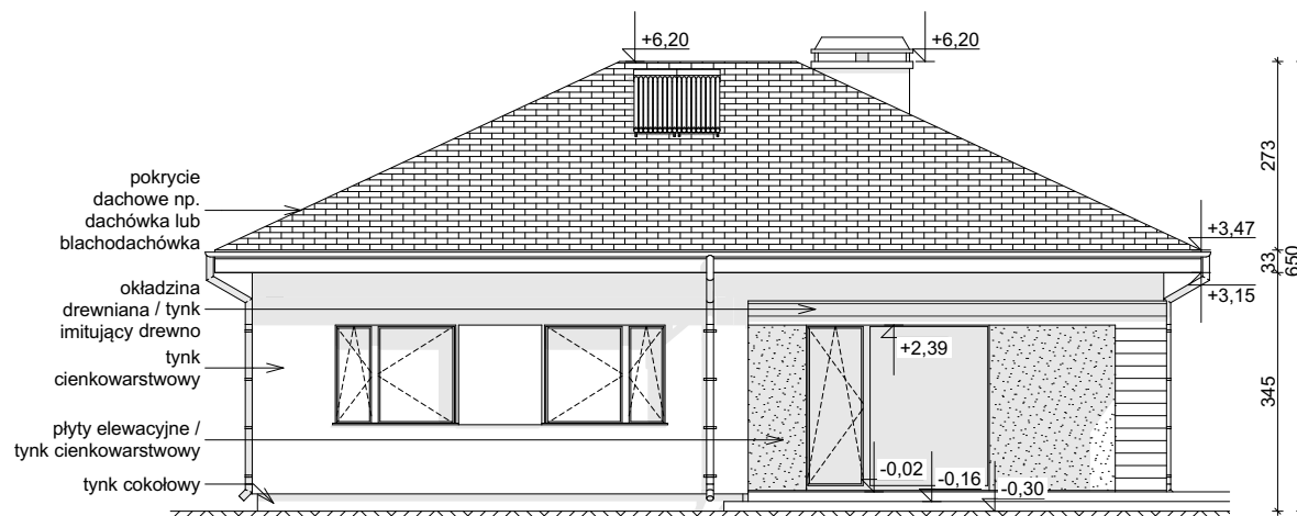
ELEWACJA OGRODOWA
