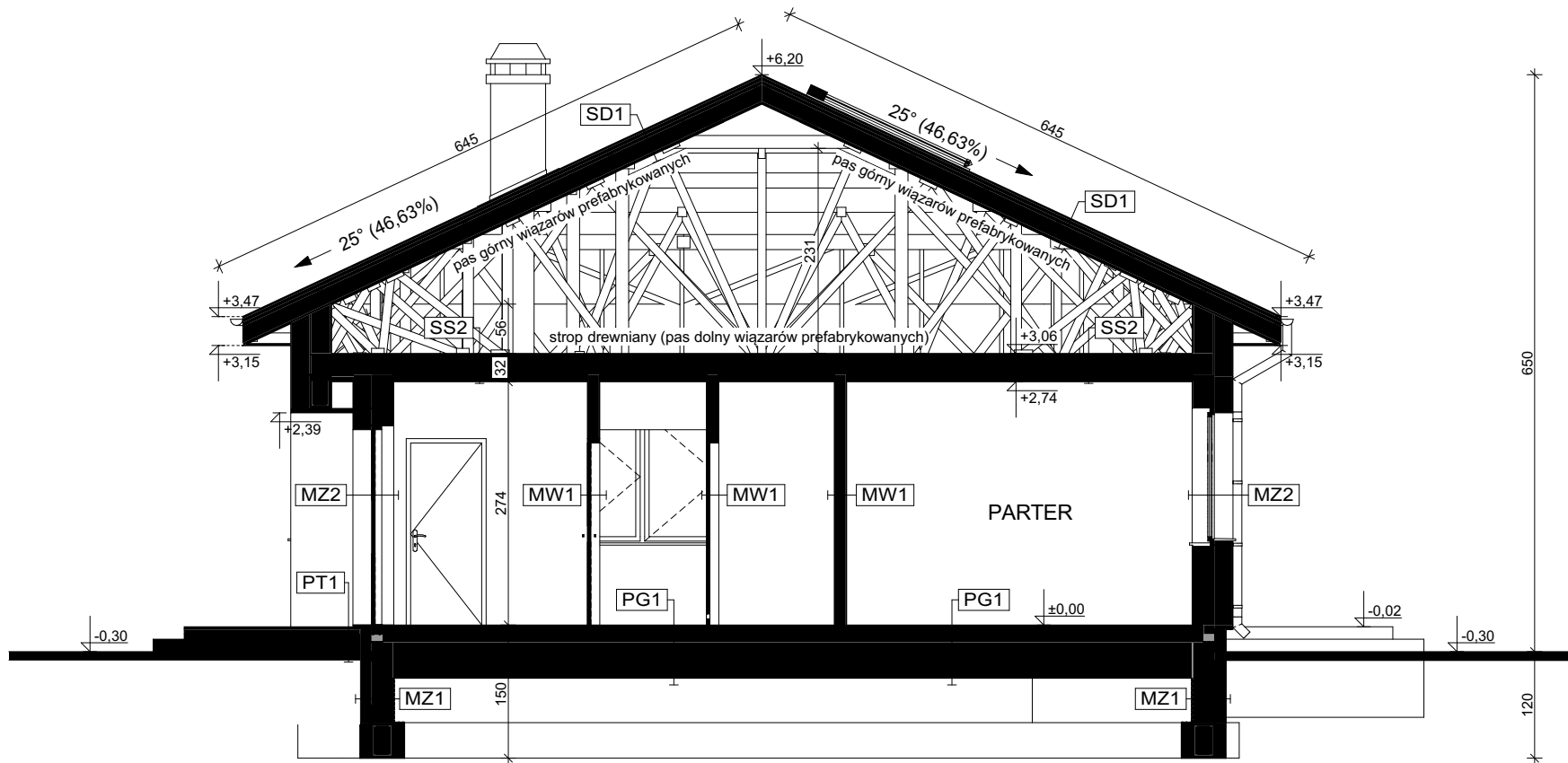
PRZEKRÓJ B-B
