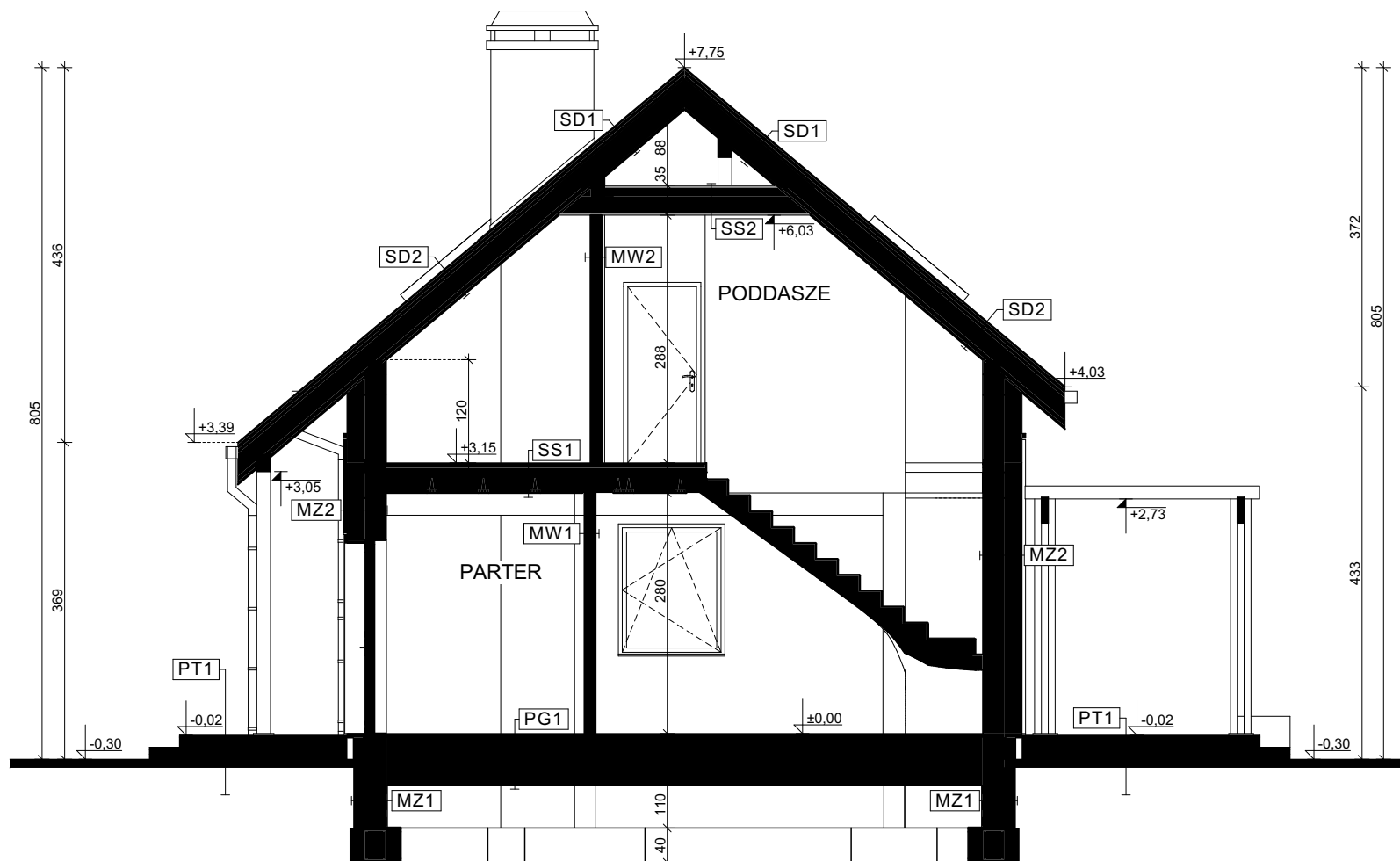
PRZEKRÓJ B-B
