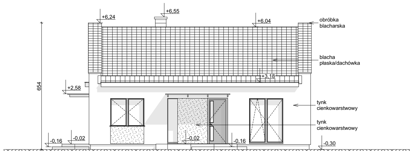
ELEWACJA FRONTOWA
