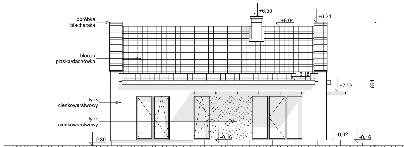
ELEWACJA OGRODOWA
