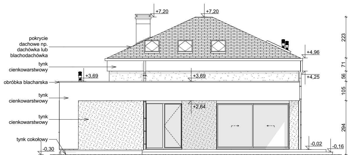
ELEVACJA BOCZNA
