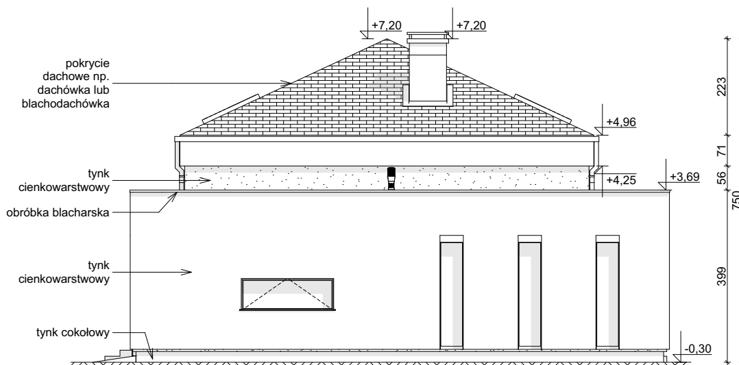
ELEVACJA BOCZNA
