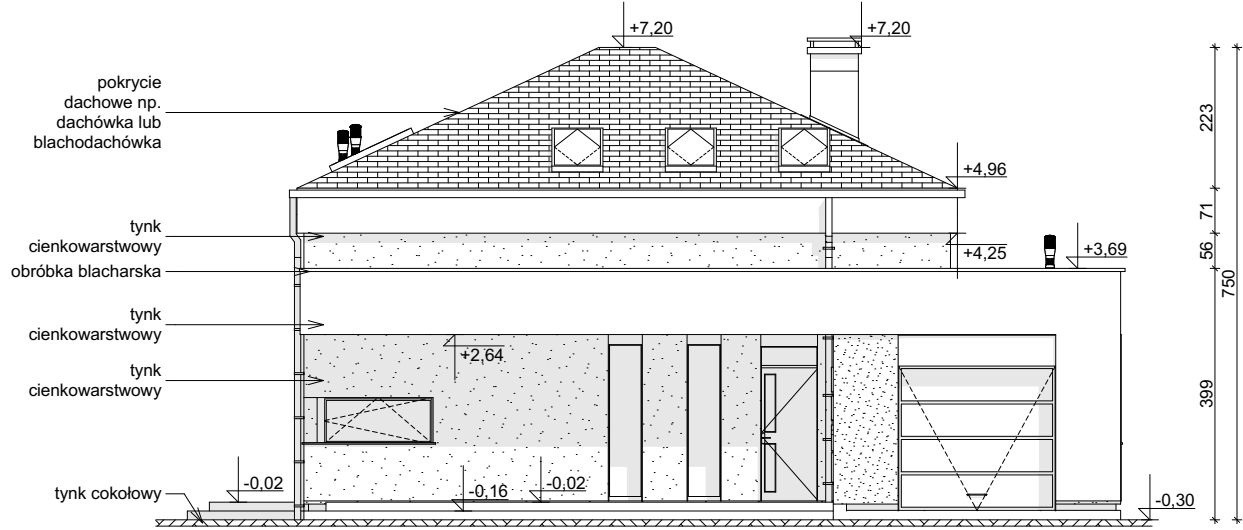
ELEWACJA FRONTOWA
