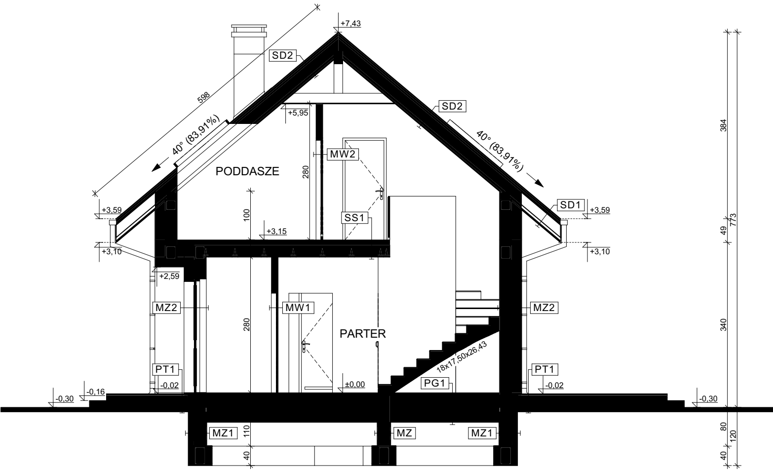
PRZEKRÓJ B-B
