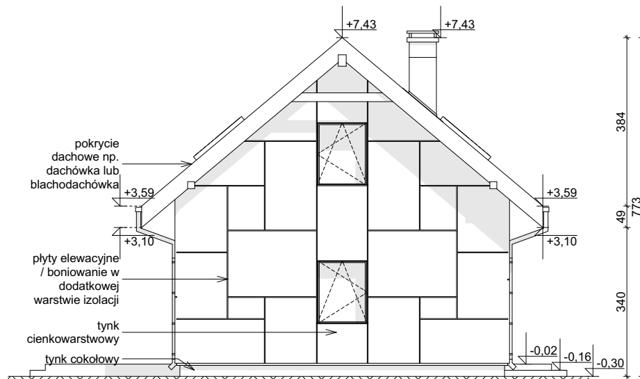
ELEWACJA BOCZNA
