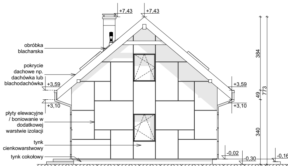
ELEWACJA BOCZNA
