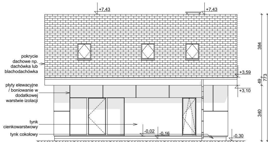
ELEWACJA OGRODOWA
