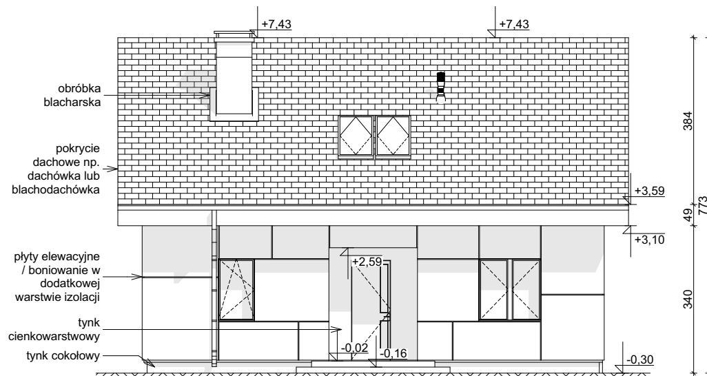
ELEWACJA FRONTOWA
