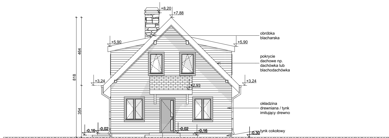
ELEWACJA FRONTOWA
