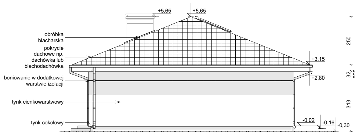
ELEWACJA BOCZNA
