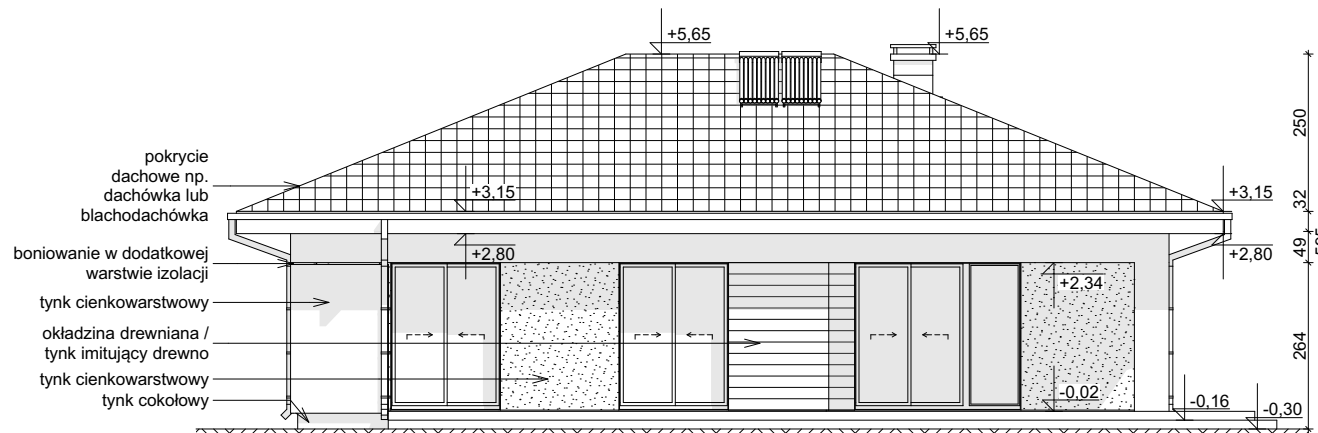
ELEWACJA OGRODOWA
