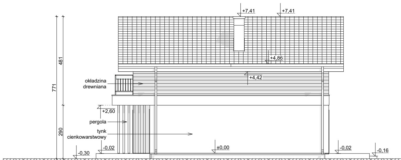
ELEVACJA BOCZNA
