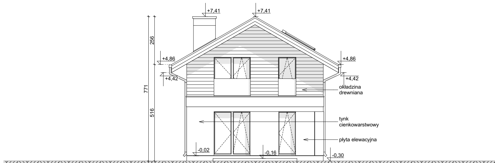
ELEVACJA OGRODOWA
