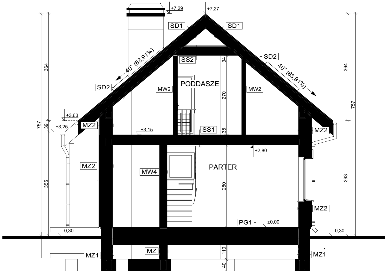
PRZEKRÓJ B-B
