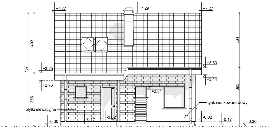
ELEWACJA FRONTOWA
