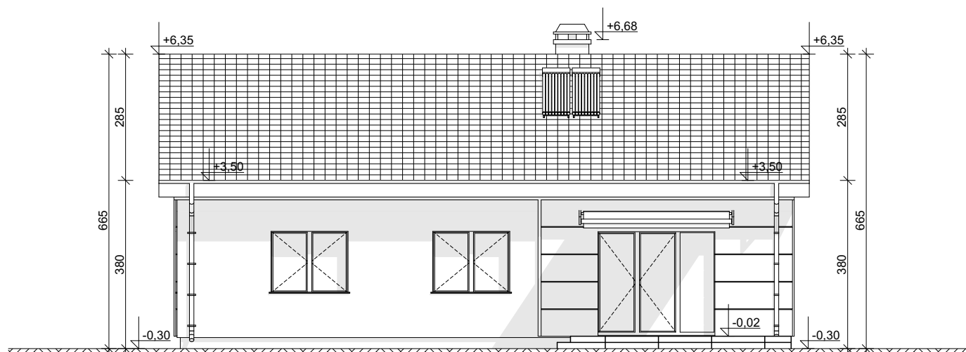
ELEWACJA OGRODOWA
