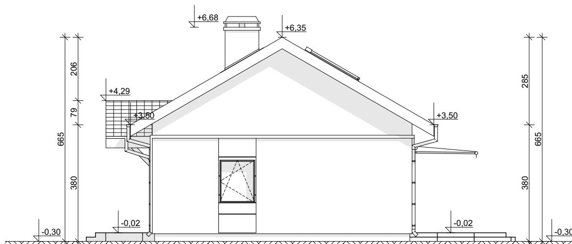
ELEWACJA BOCZNA
