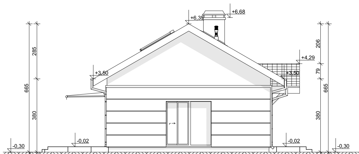
ELEWACJA BOCZNA
