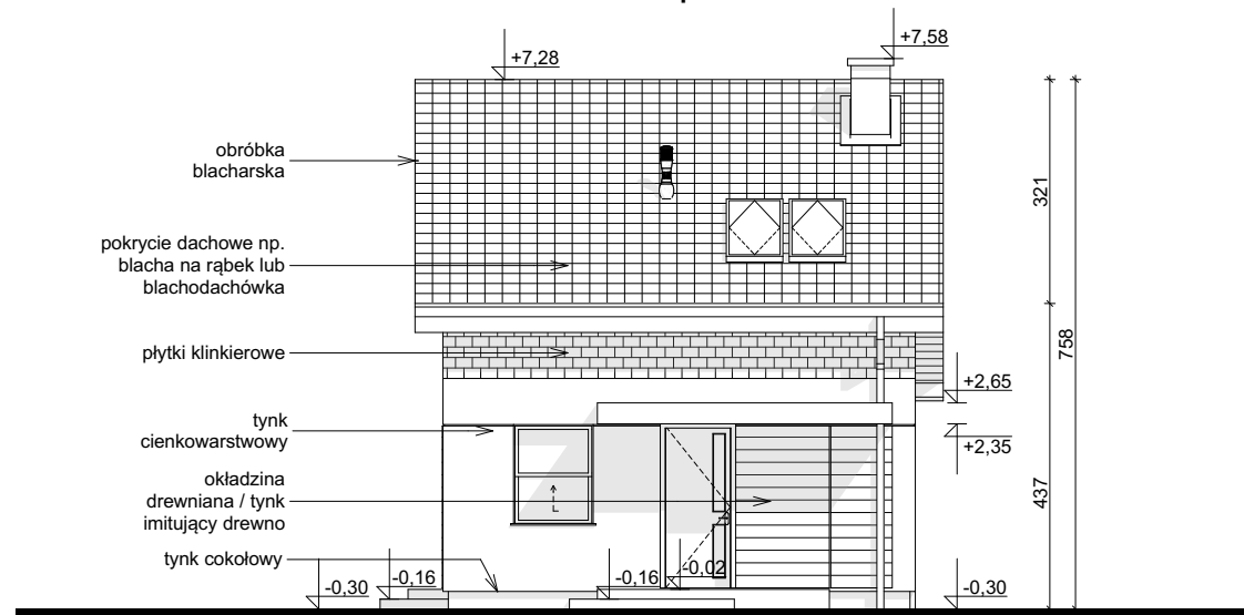
ELEWACJA FRONTOWA
