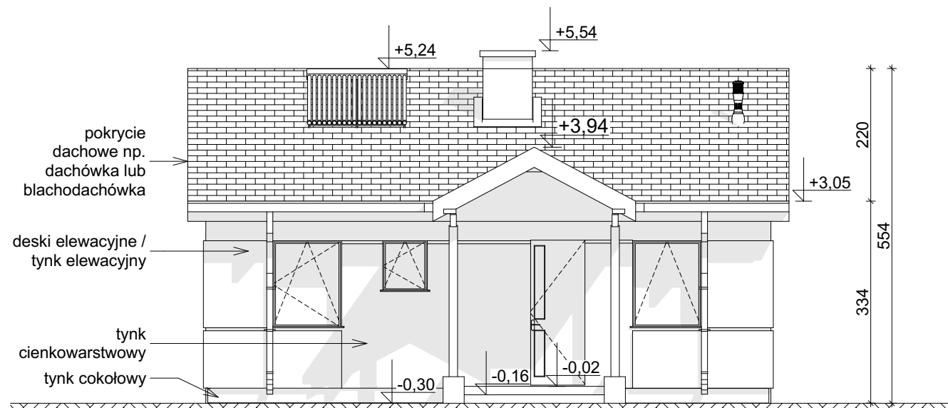
ELEWACJA FRONTOWA
