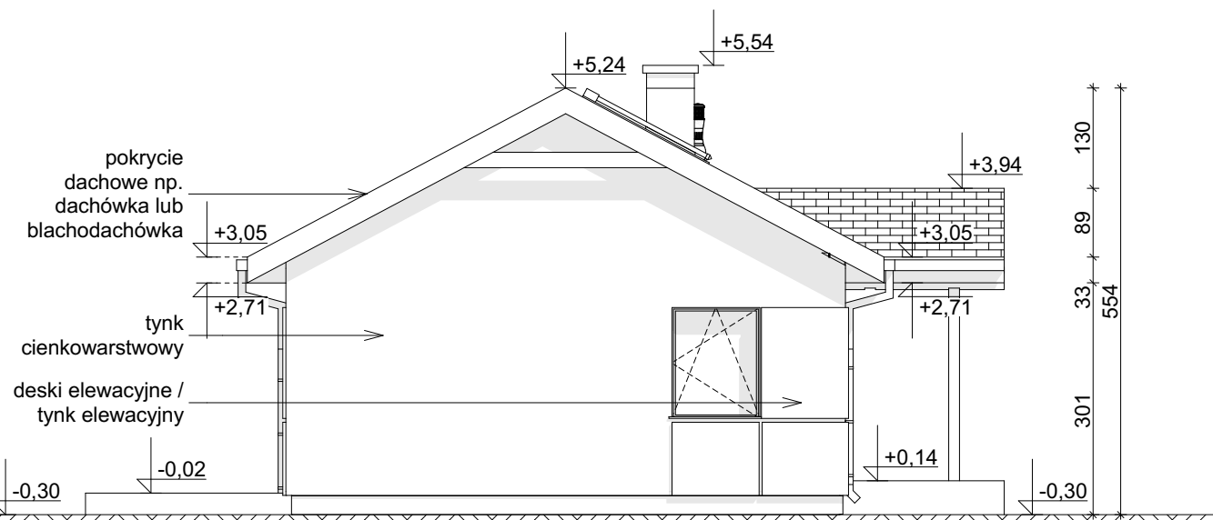
ELEWACJA BOCZNA
