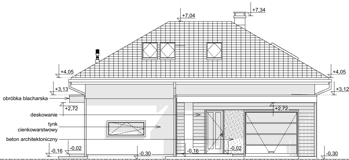
ELEWACJA FRONTOWA
