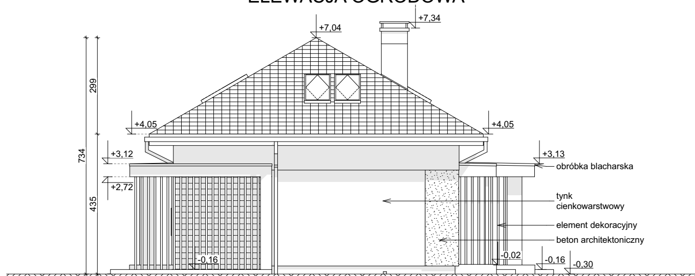
ELEWACJA BOCZNA
