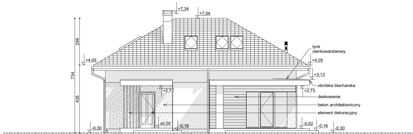
ELEWACJA OGRODOWA
