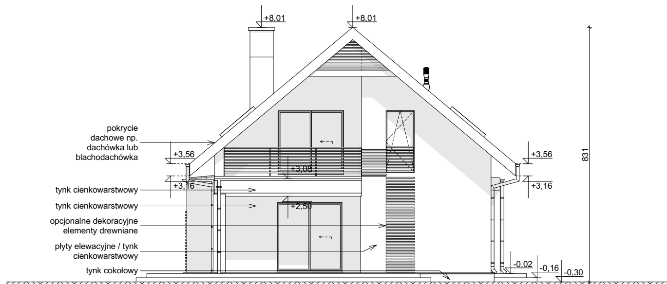
ELEWACJA BOCZNA
