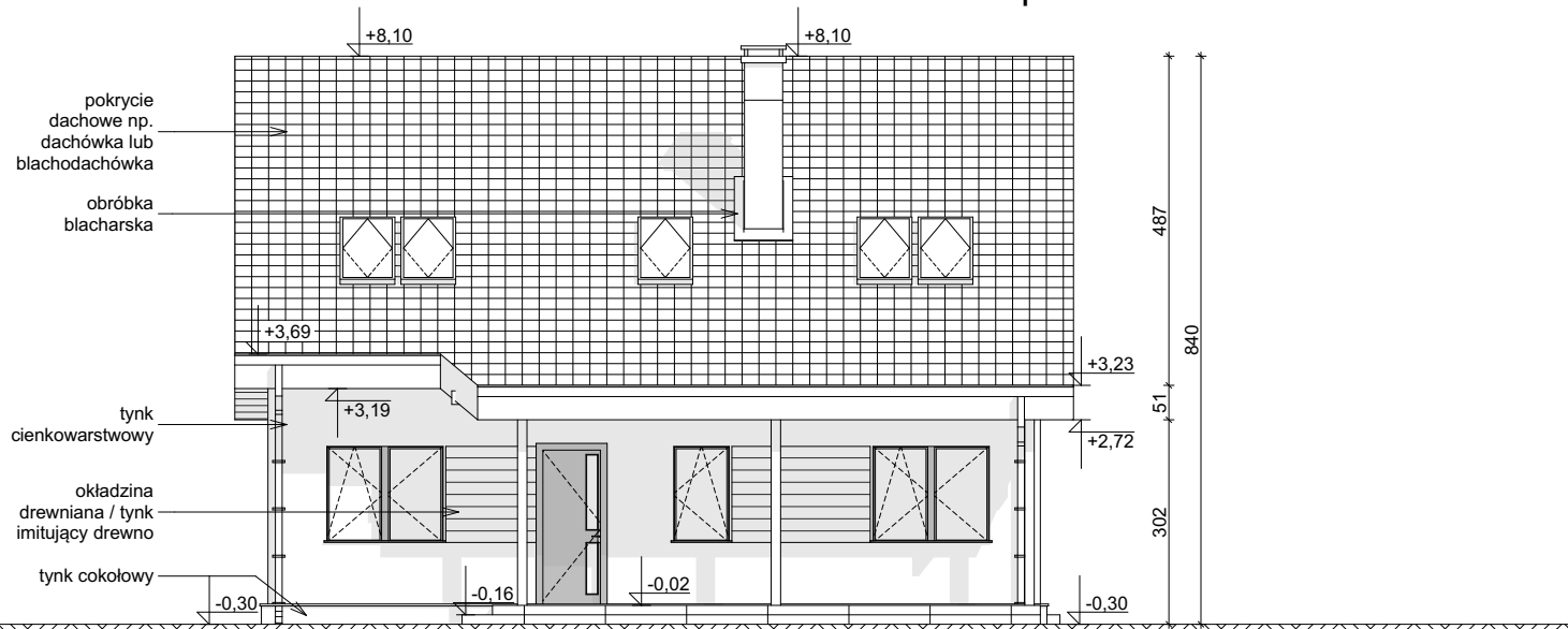
ELEWACJA FRONTOWA
