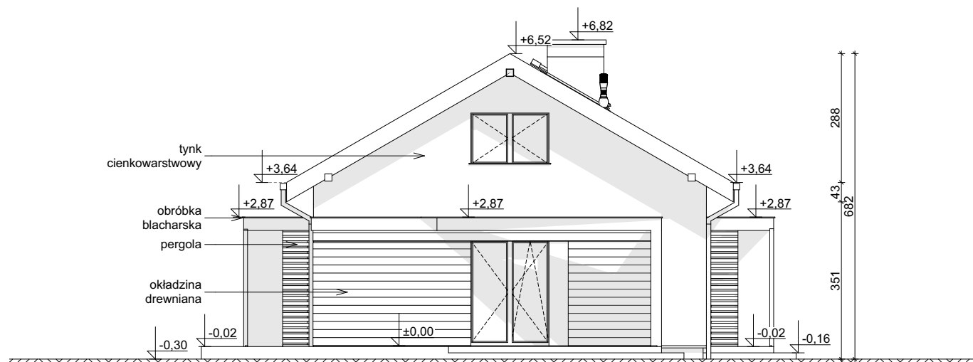
ELEWACJA BOCZNA
