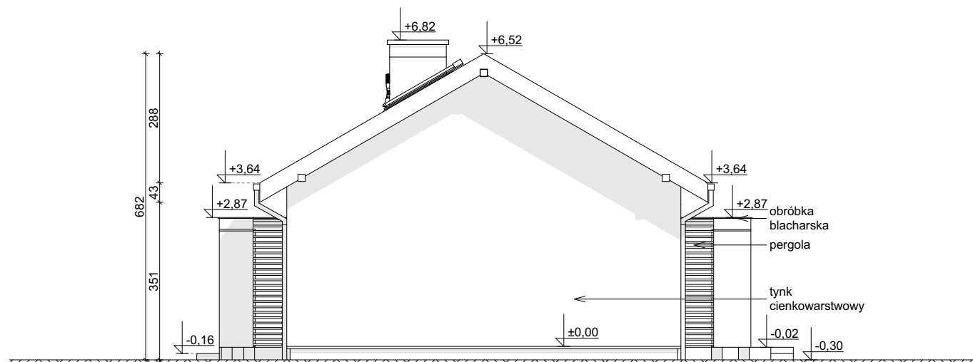
ELEWACJA BOCZNA
