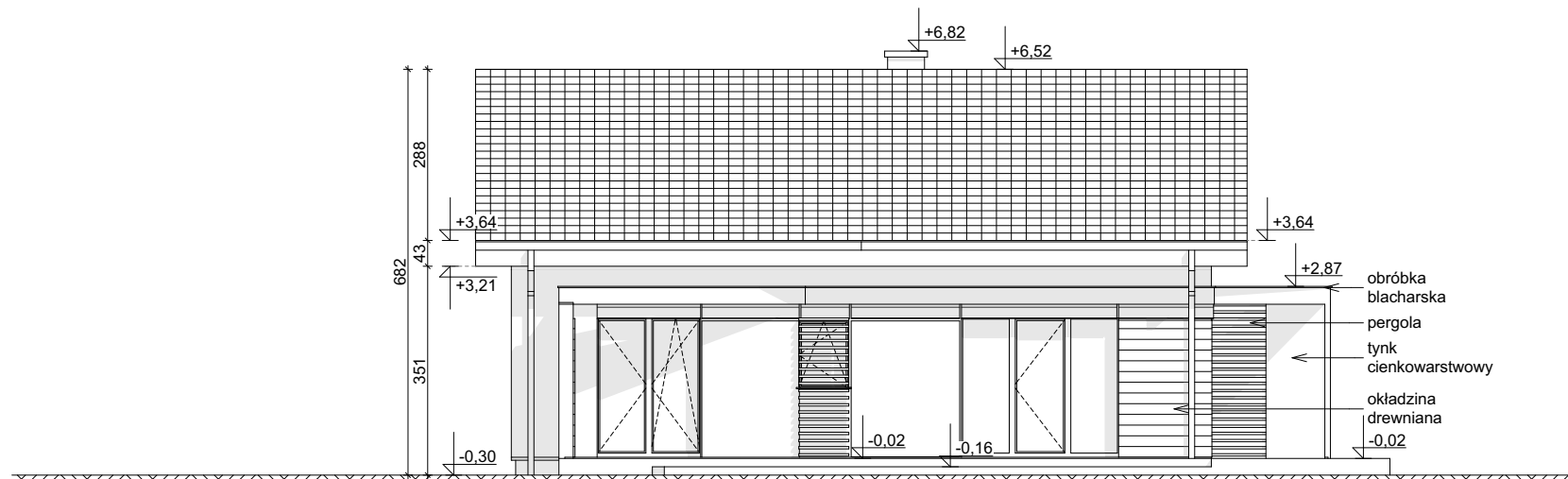
ELEWACJA OGRODOWA
