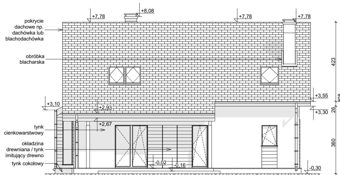
ELEWACJA OGRODOWA
