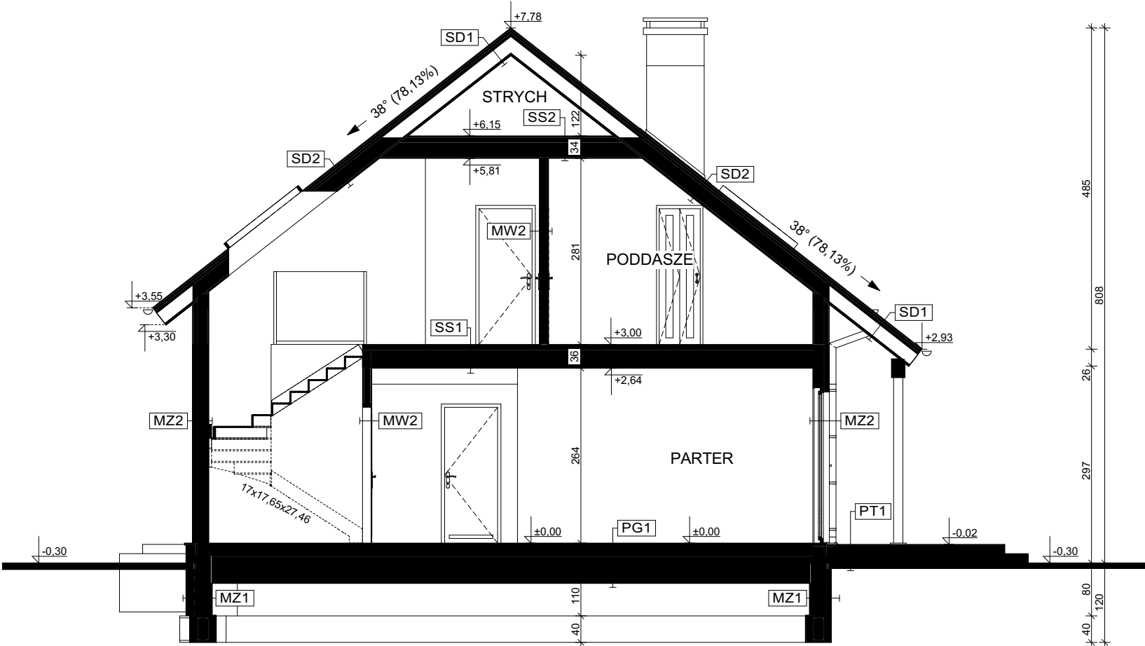
PRZEKRÓJ B-B
