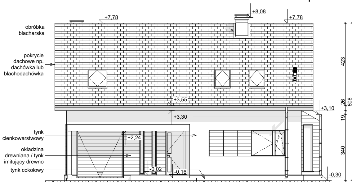
ELEWACJA FRONTOWA
