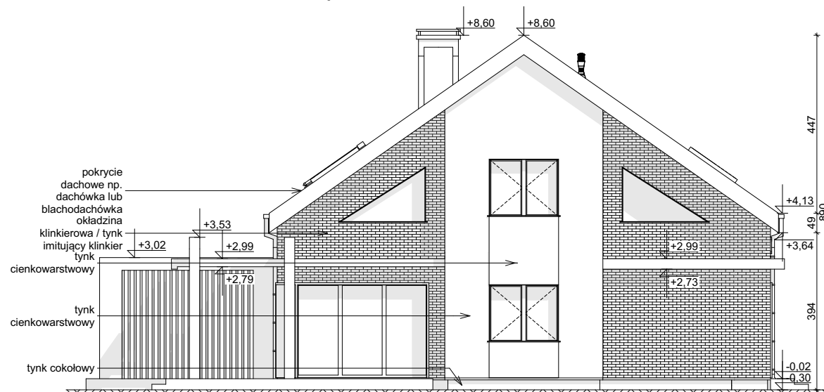
ELEWACJA BOCZNA
