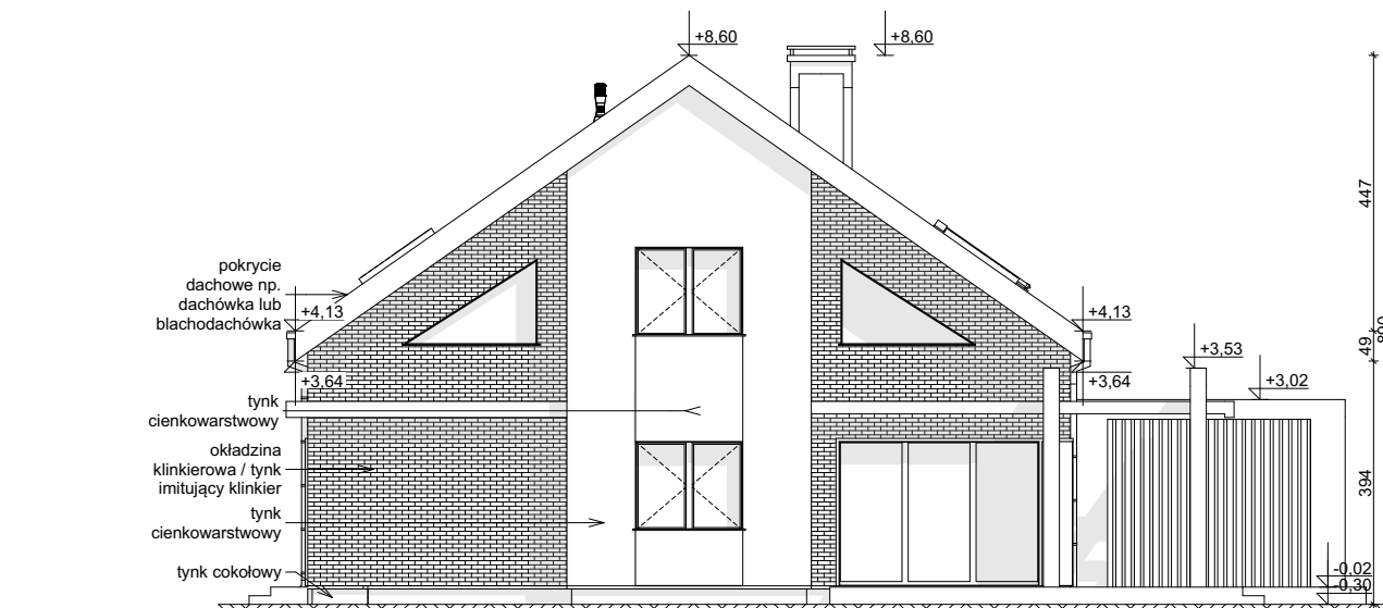
ELEWACJA BOCZNA
