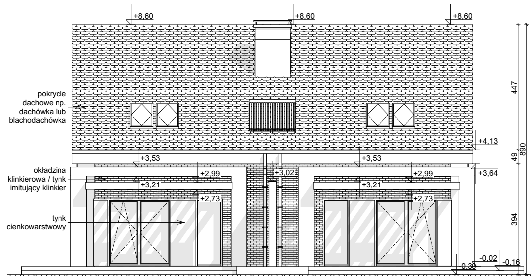
ELEWACJA OGRODOWA
